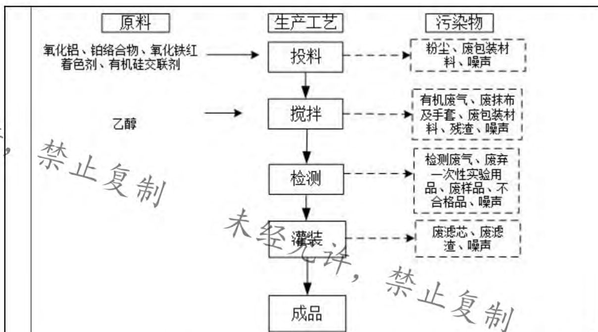
图 2-5 导热胶生产工艺流程及产污节点图
