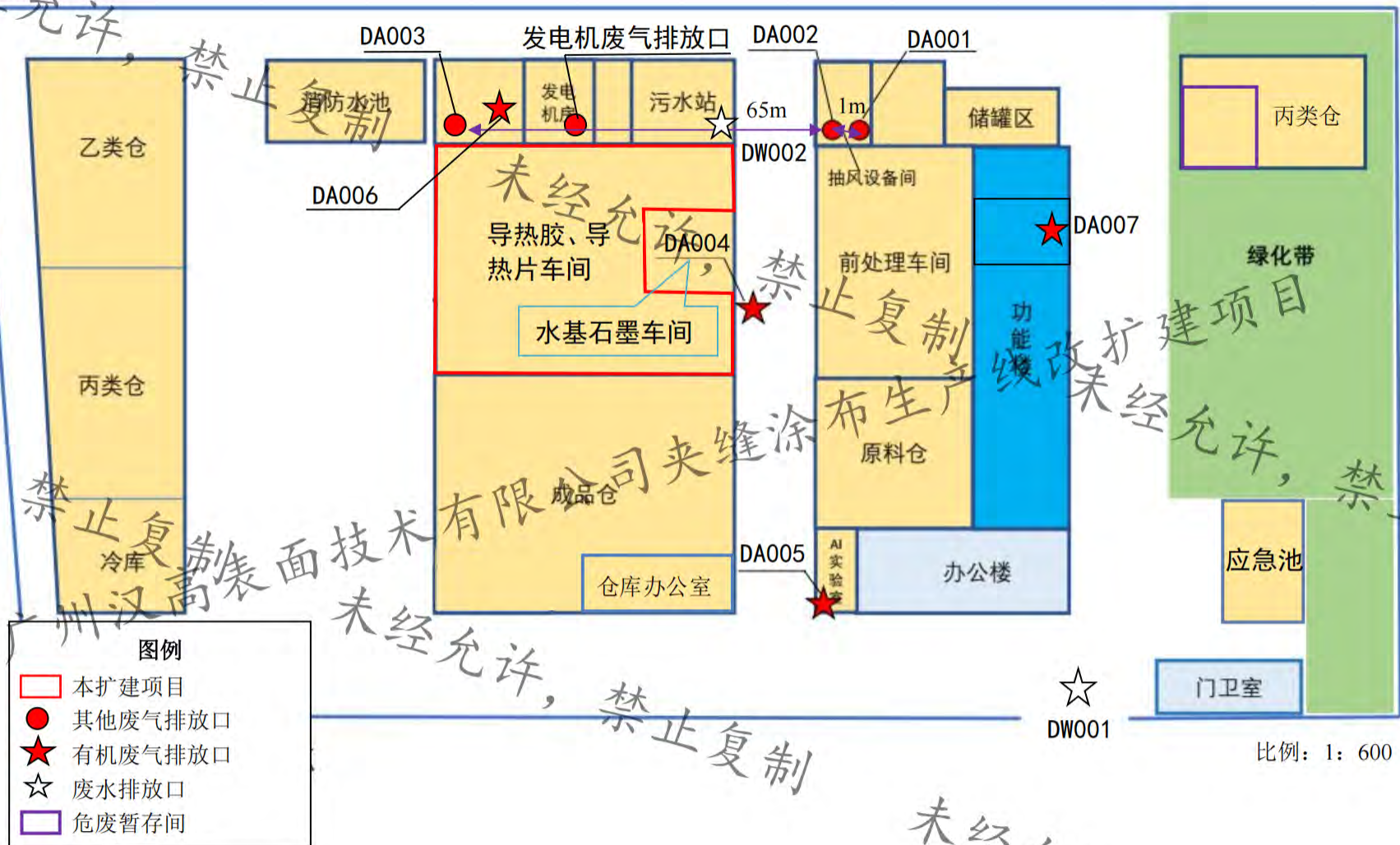
附图 2-1 厂区总平面布置图
