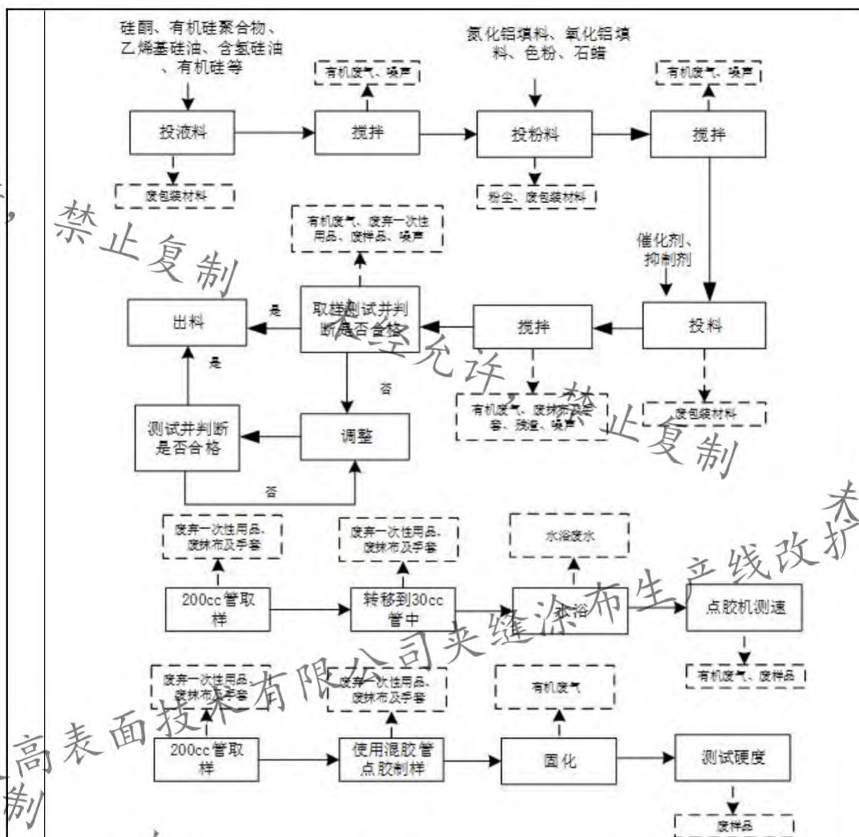
图2-14 导热产品研发工艺流程及产污节点图
