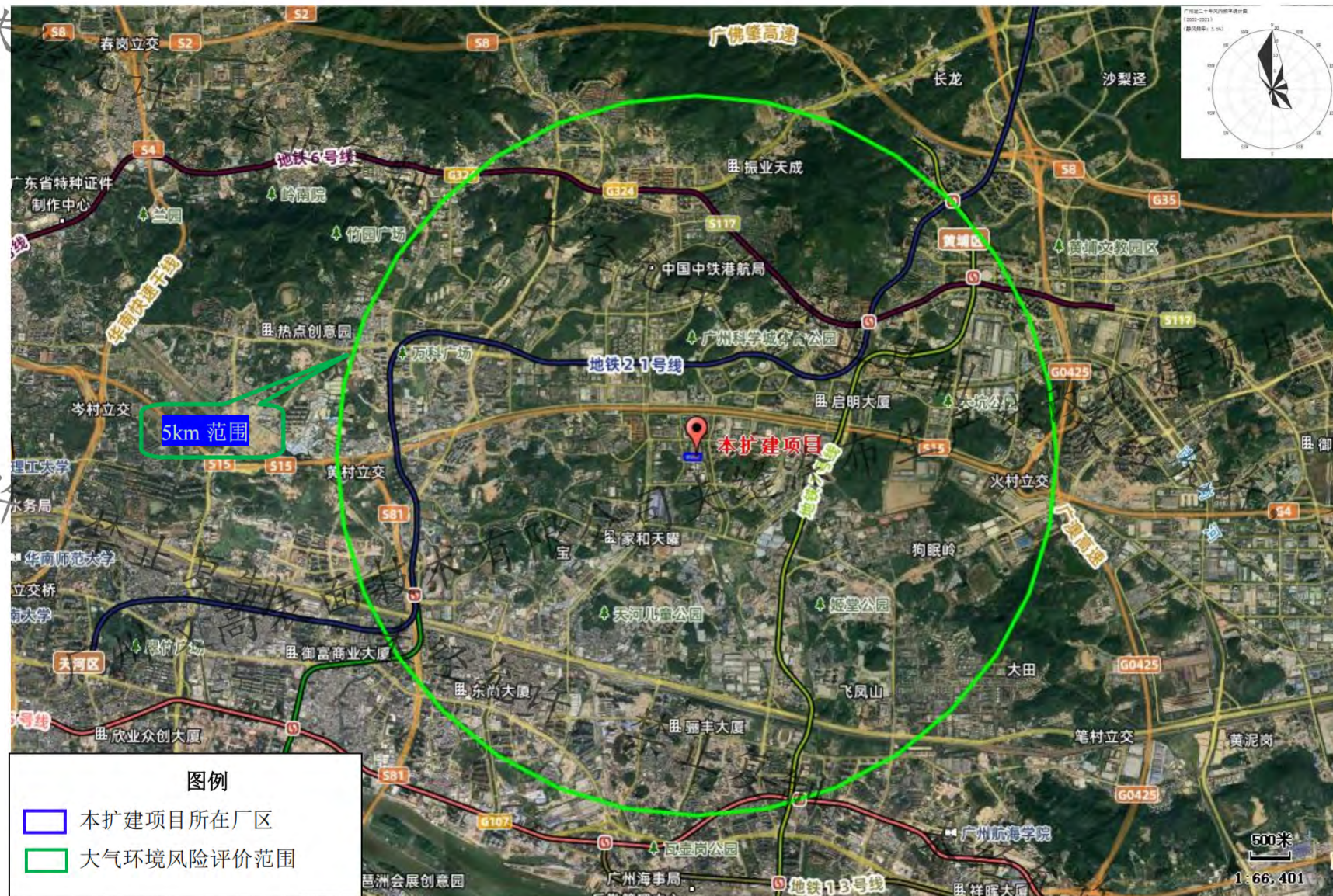
图 2.3-1 项目环境风险评价范围图
