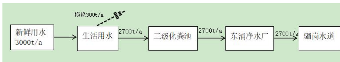
图 2-2 本项目水平衡图 (t/a)
