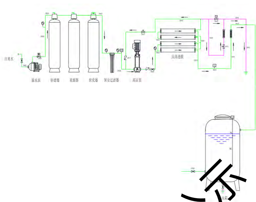
图 4.2-10 纯水制备工艺流程
