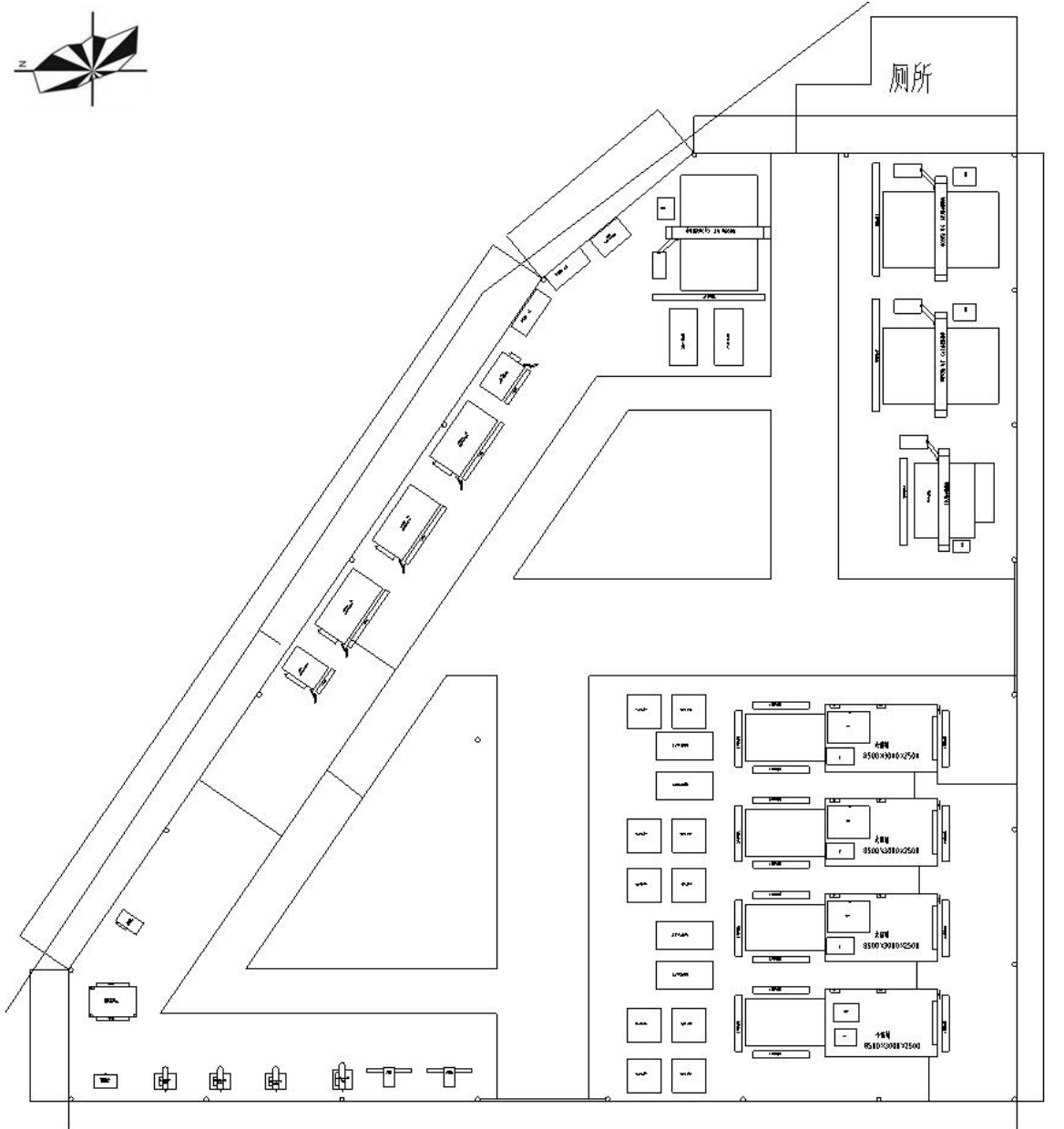
附图 4-3：冲压钣金车间
