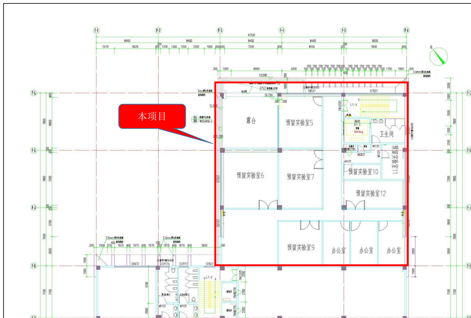
附图 5-2：建设项目平面布局图（三楼）
