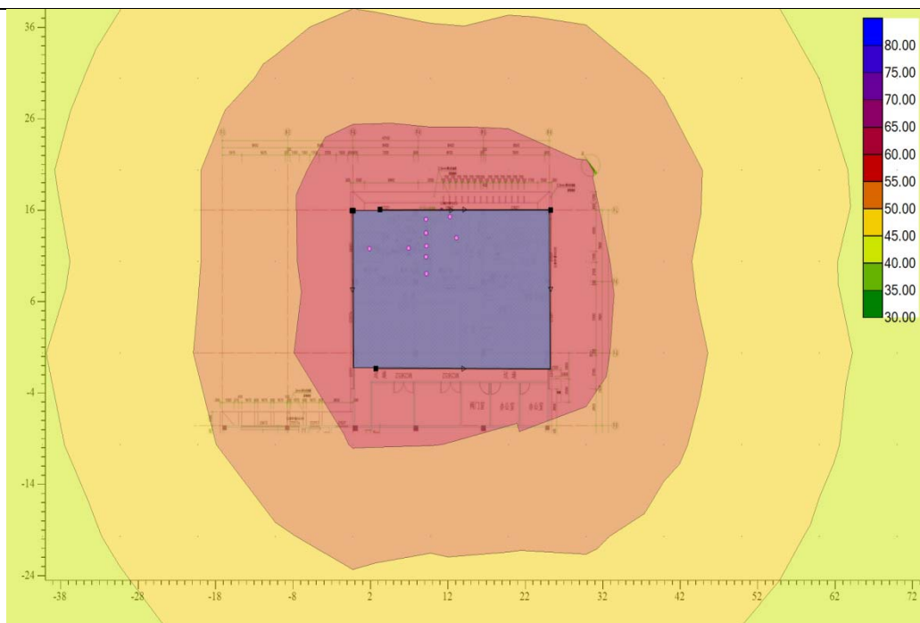
图 4.2.3-1 项目实验设备运行等声值线图
