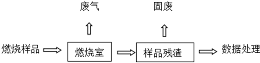
图 2.4-7 纺织品垂直燃烧试验工艺流程图
