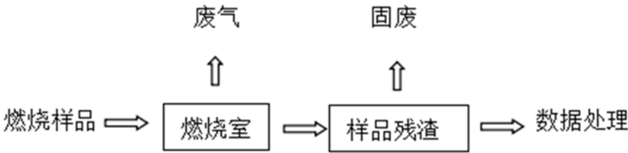
图 2.4-5 分解烟密度试验工艺流程图
