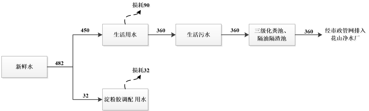
图 2-1 项目全厂总水平衡图 \text{m}^3/\text{a}
