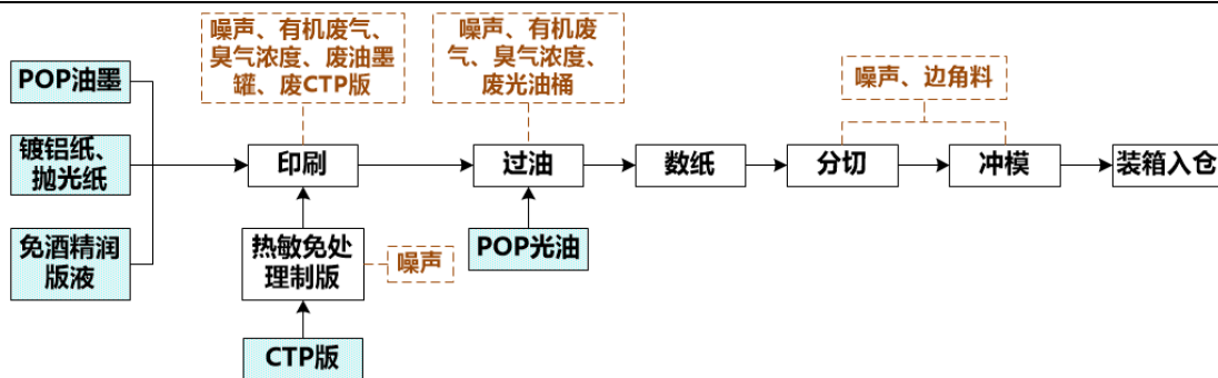
图2-5 商标生产工艺流程图
