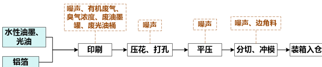
图2-6 铝帽生产工艺流程图
