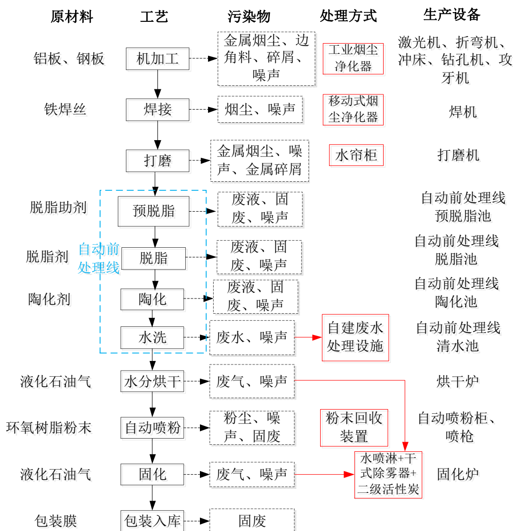
图 3 项目方板生产工艺流程图
