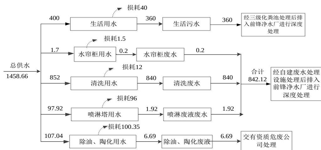
图 2 项目水平衡图 单位: \text{m}^3/\text{a}
