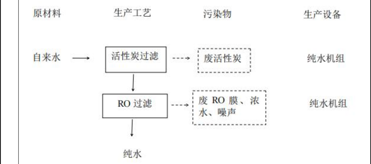
图 2-15 纯水制备工艺流程图
