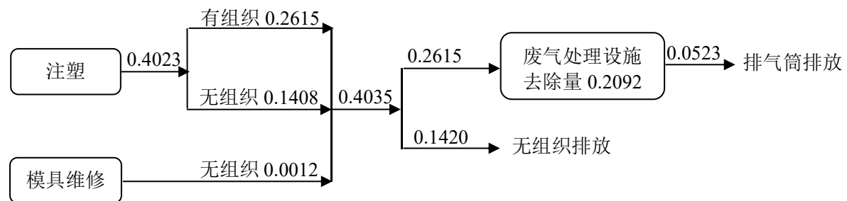
图 4-2 VOCs 平衡图 单位 t/a
