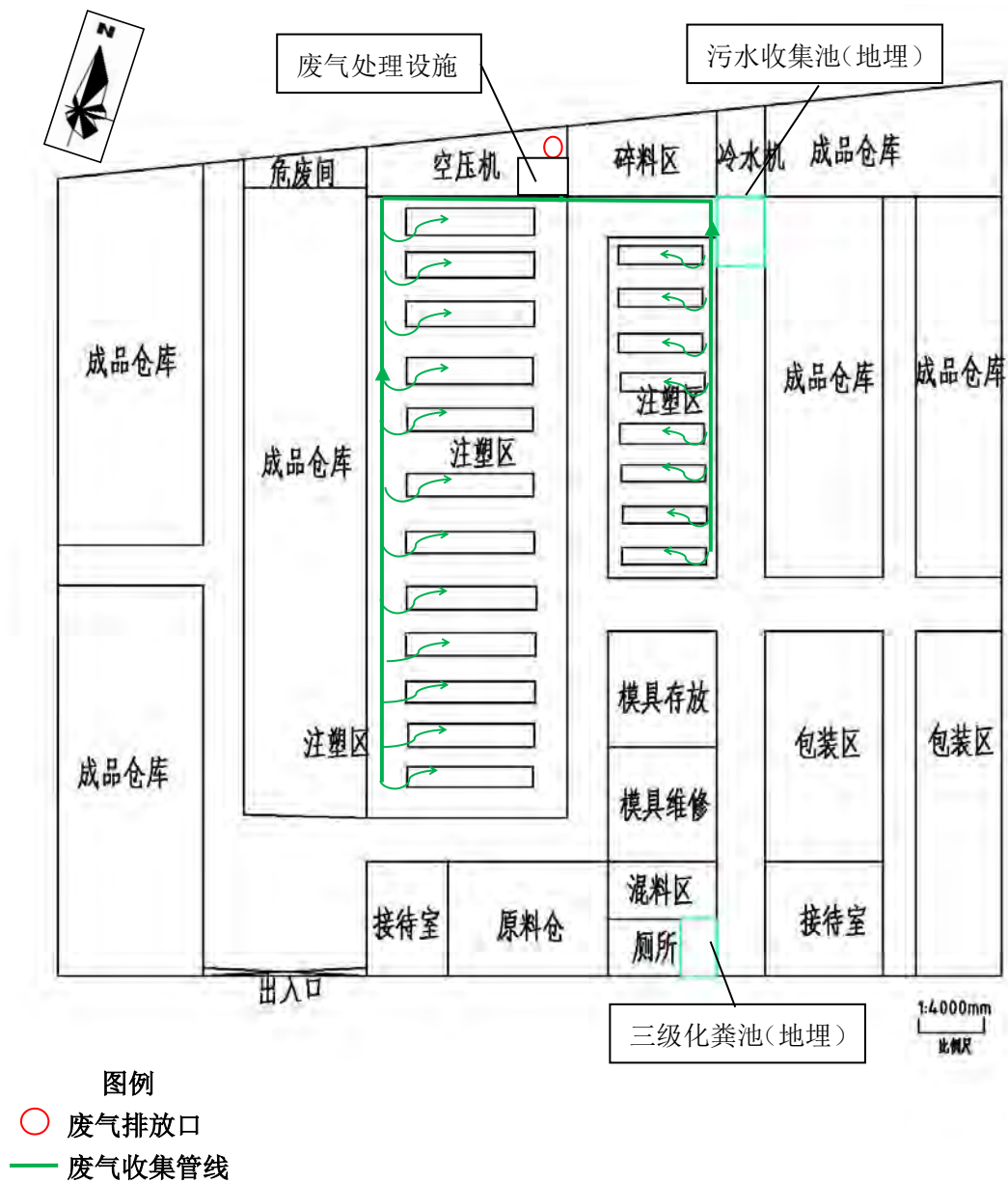
附图 5 项目厂区平面布置图
