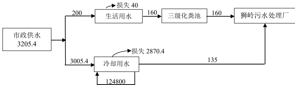
图 2-2 全厂远期水平衡图 (单位: m³/a)
