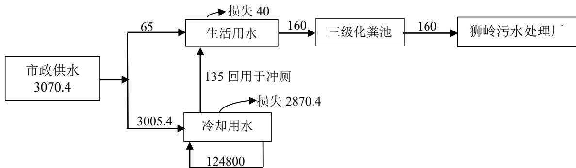
图 2-1 全厂近期水平衡图 (单位: m³/a)
