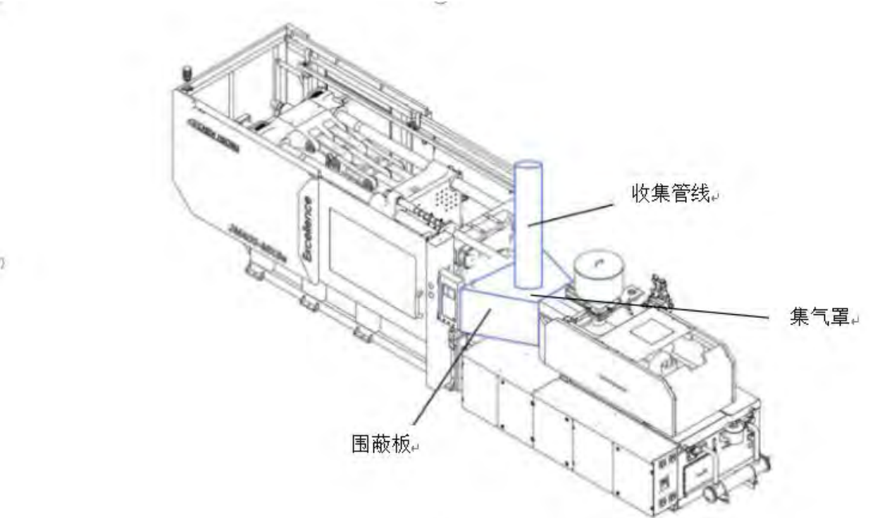
图 4-1 废气收集示意图
