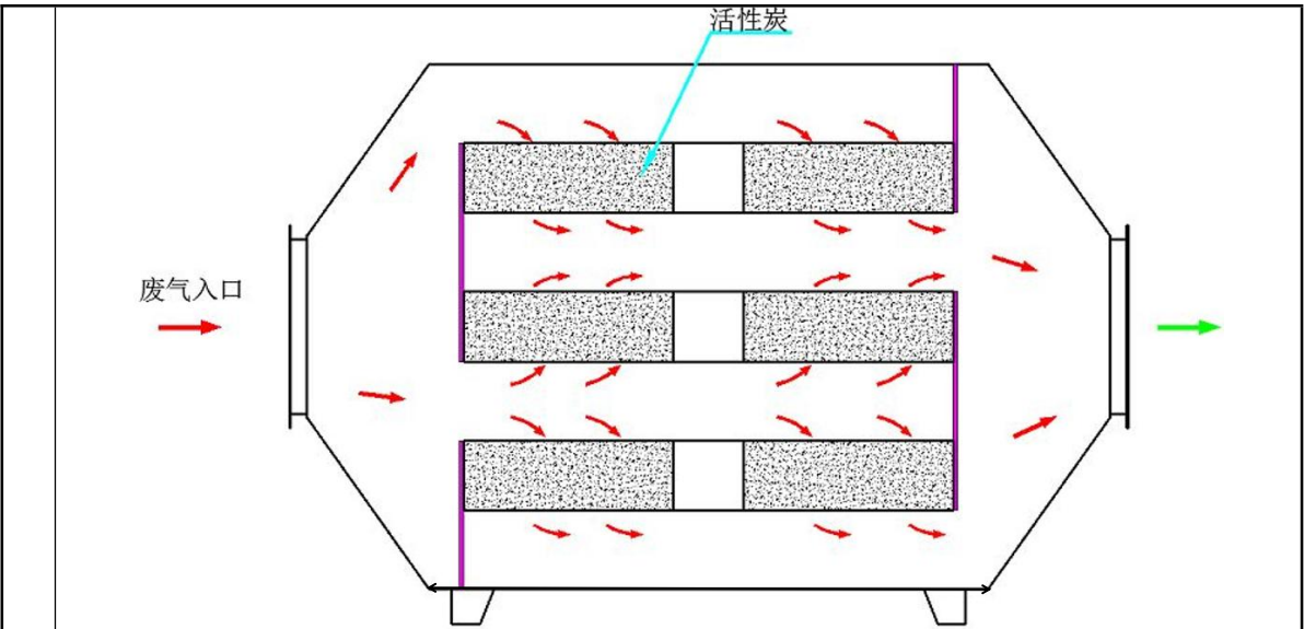
图 4-1 本项目活性炭箱设计图
