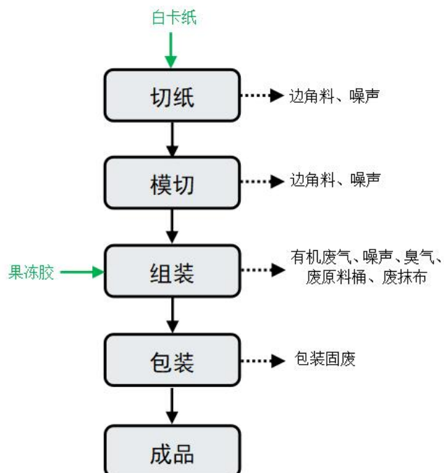
图 2-3 化妆品精装盒生产工艺流程及产污环节图
