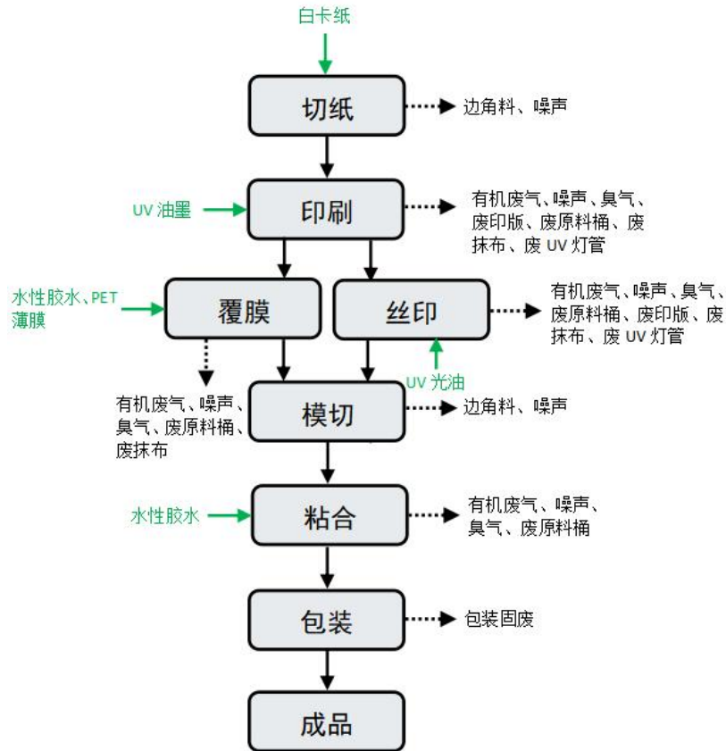
图 2-2 化妆品彩盒生产工艺流程及产污环节图
