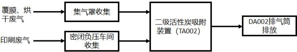
图 4-2.2 2#厂房废气处理工艺图
