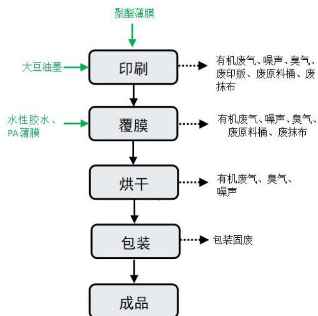
图 2-4 印刷薄膜生产工艺流程及产污环节图
