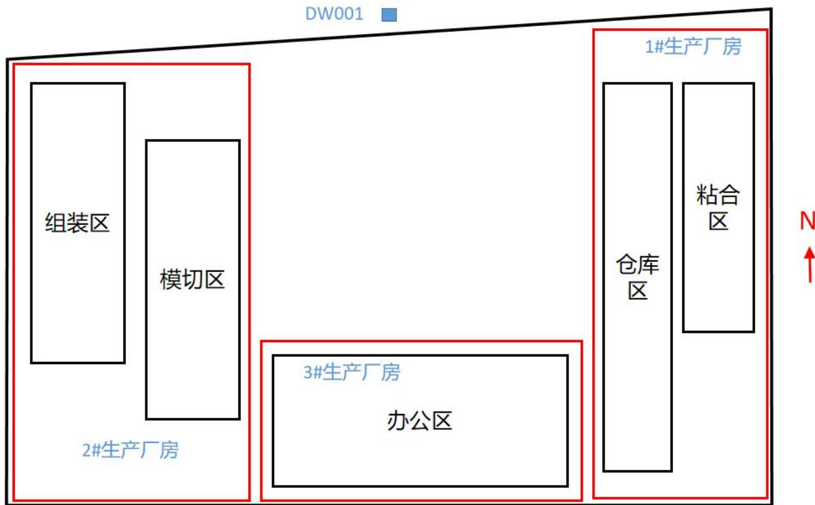
附图 3.3 项目车间二楼布置平面图
