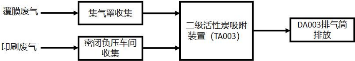
图 4-2.3 3#厂房废气处理工艺图
