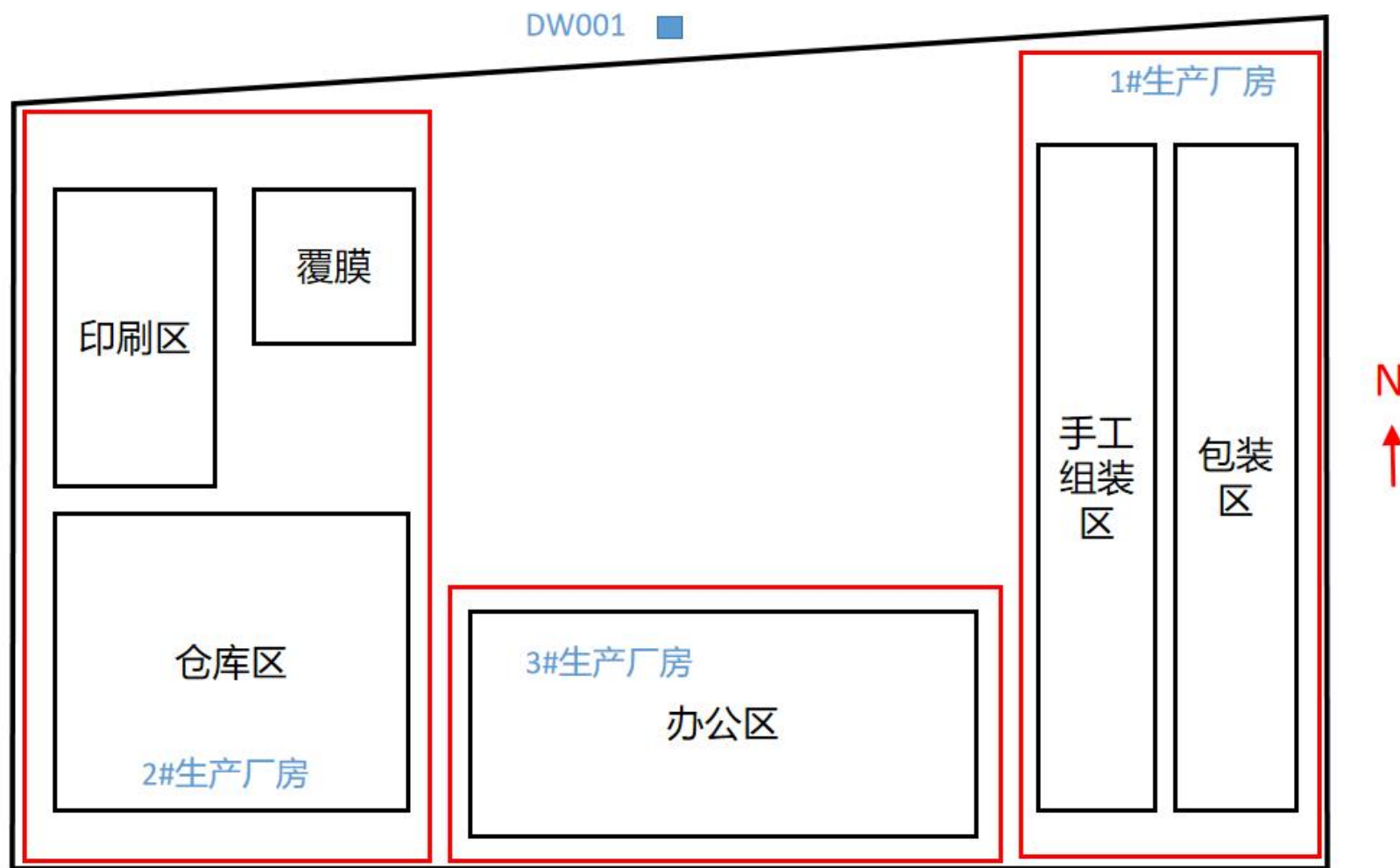
附图 3.4 项目车间三楼布置平面图
