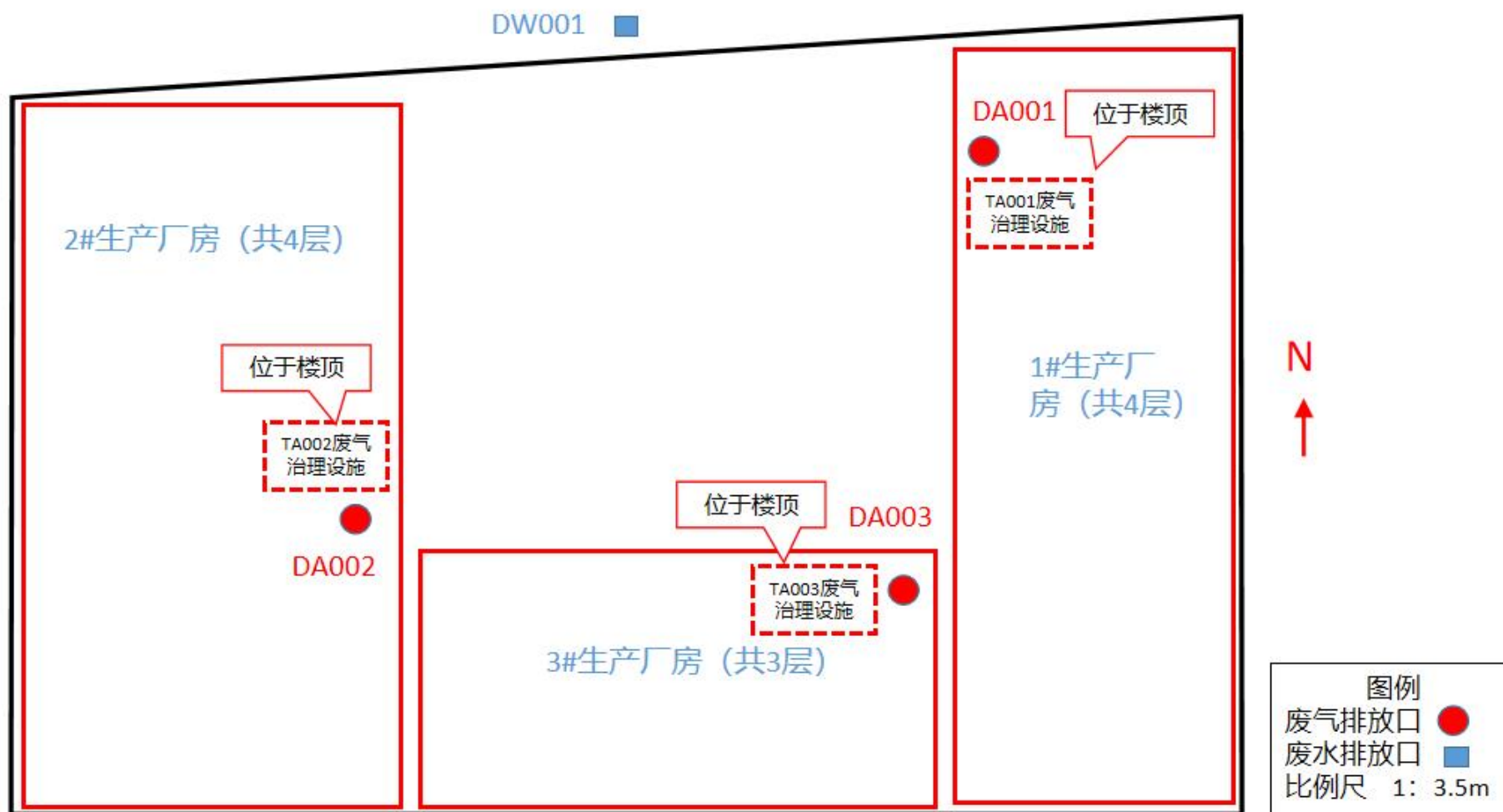
附图 3.1 项目厂区布置平面图
