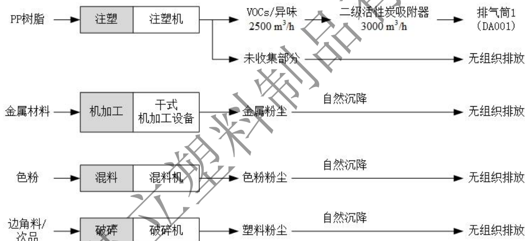
图 4-2 废气收集、治理和排放汇总示意图
