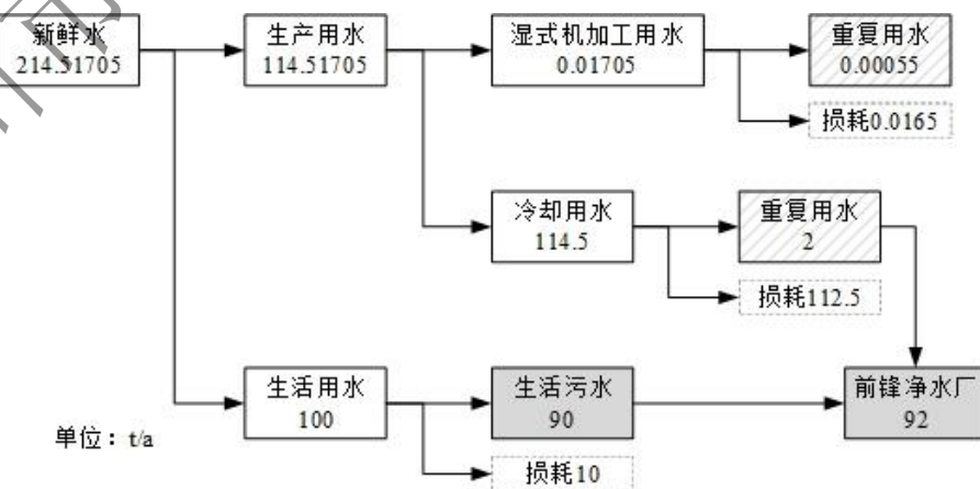
图 2-1 水平衡示意图
