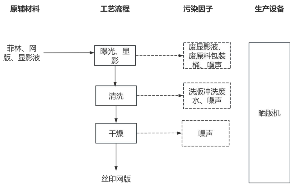
图 2-5 本项目制版工艺流程及产污环节图
