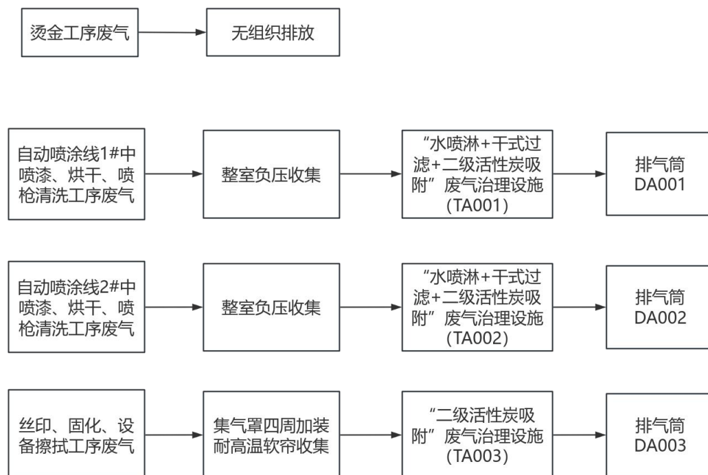
图 4-1 废气治理设施流程图
