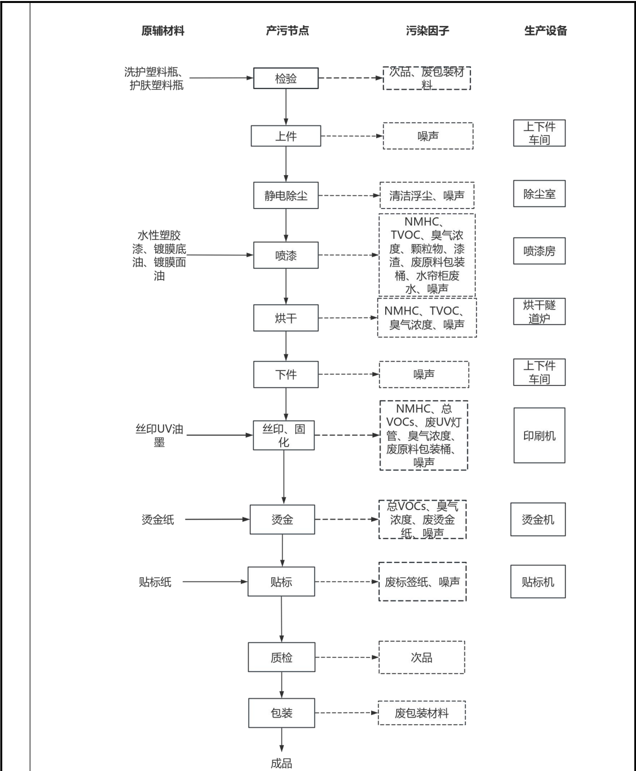
图 2-4 本项目塑料瓶工艺流程及产污环节图
