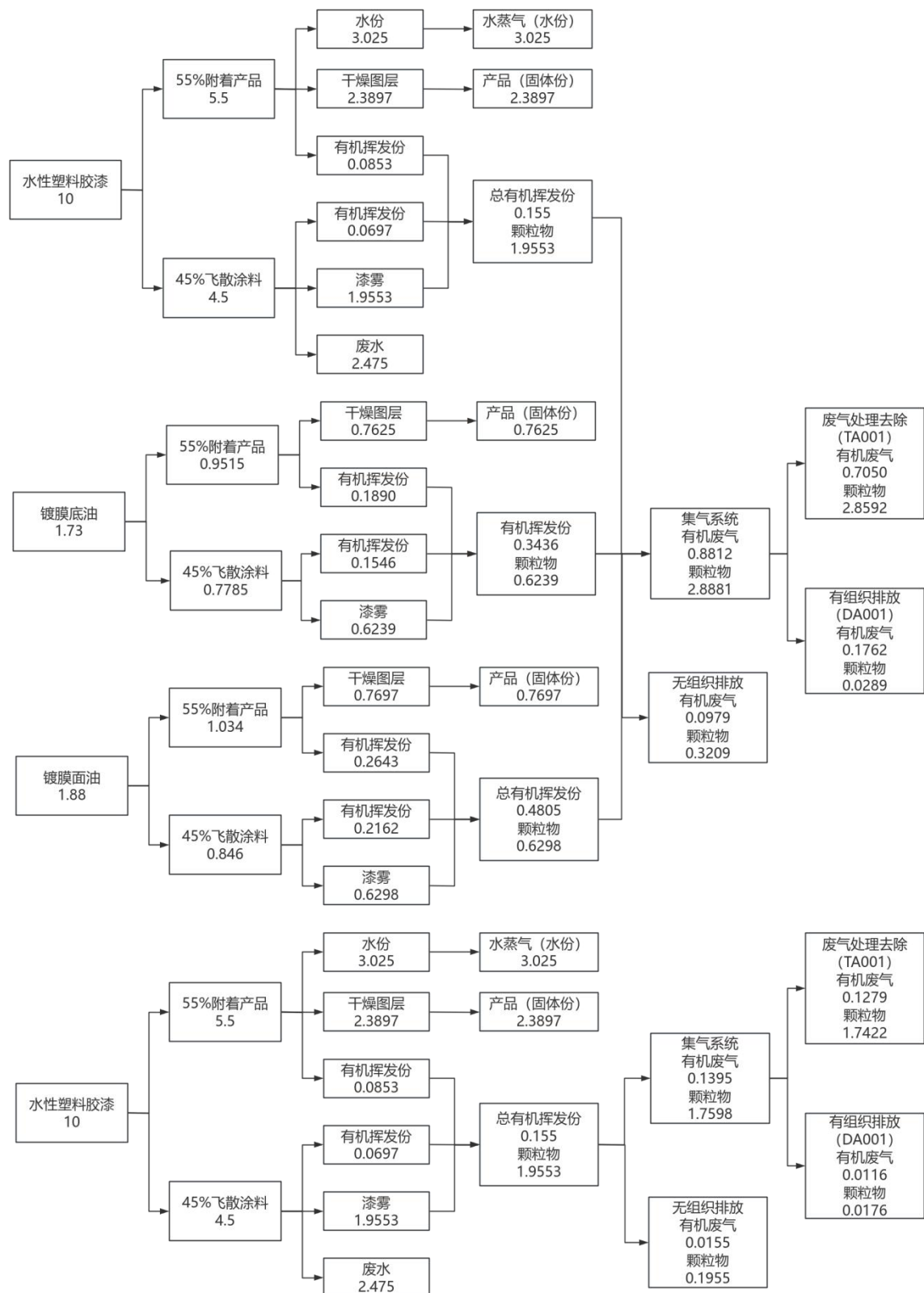
图 2-3 本项目漆料平衡图 (单位 t/a)
