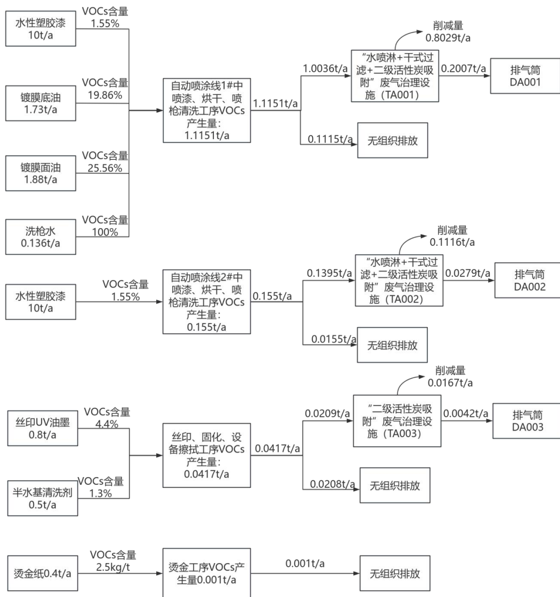
图 2-2 本项目 VOCs 平衡图
