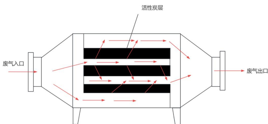
图 4-2 本项目活性炭箱设计图
