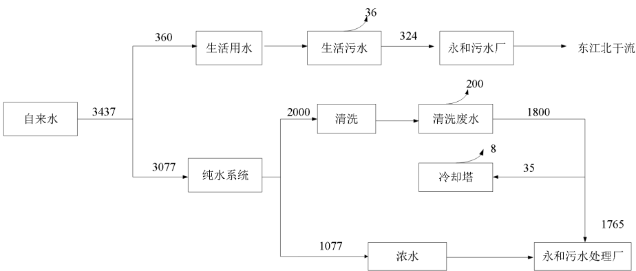
图 2-1 迁扩建前项目水平衡图 (m 3 /a)
