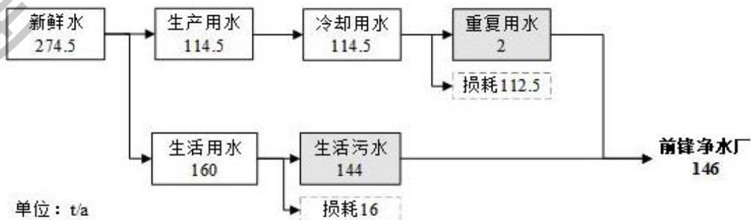
图 2-1 水平衡示意图
