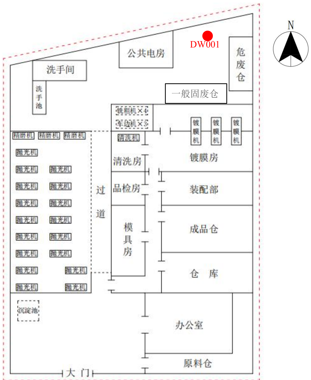
附图 4 项目平面布置图
