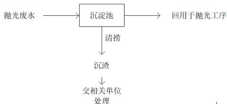
图 4-2 抛光废水处理流程
