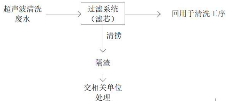
图 4-3 超声波清洗废水处理流程
