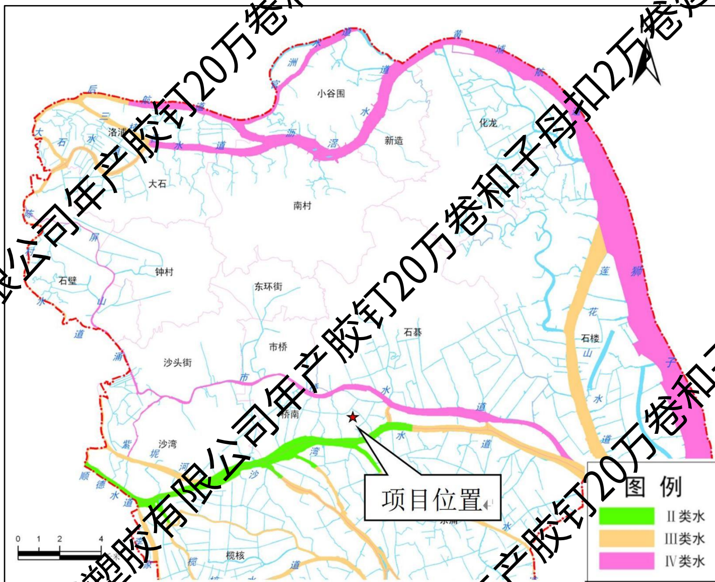
附图 5 项目所在区域水体功能区划图
