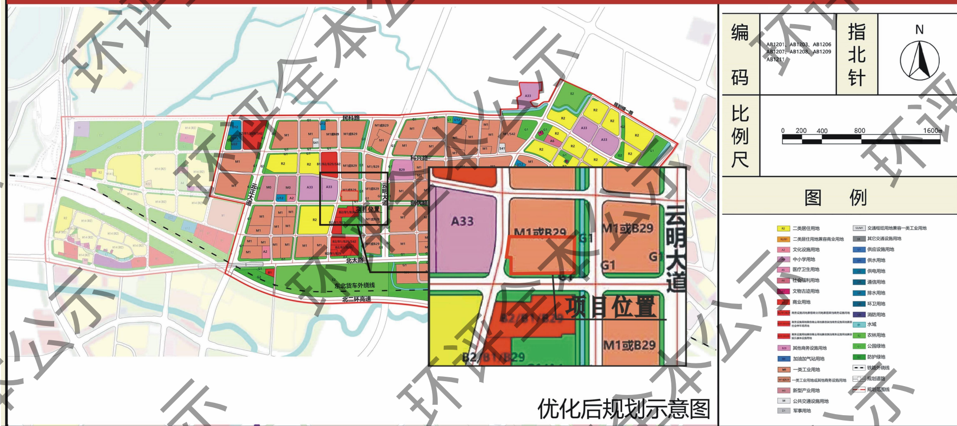
附图 21 广州民营科技园核心区控制性详细规划图
