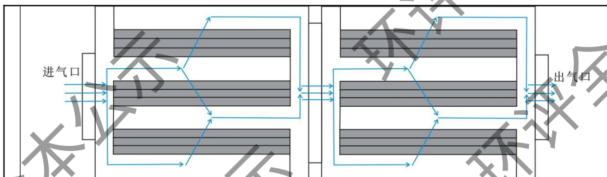
二级活性炭吸附装置工作示意图
