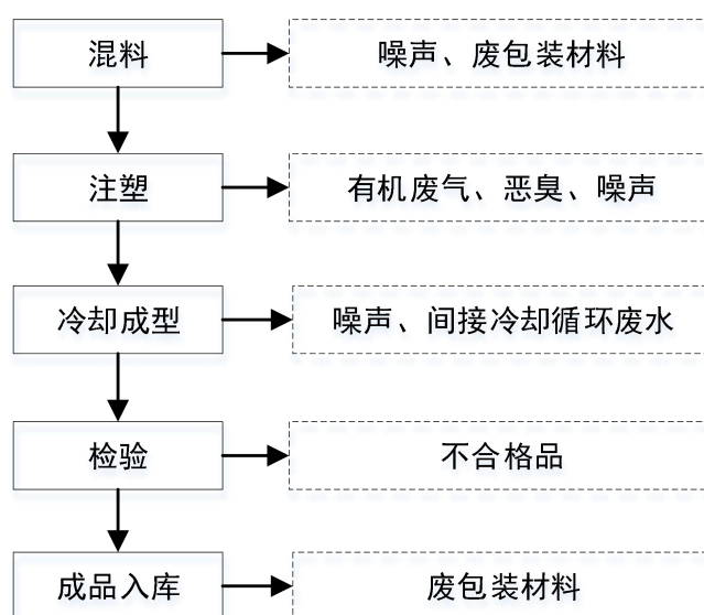
图 2-3 工艺流程及排污节点图
