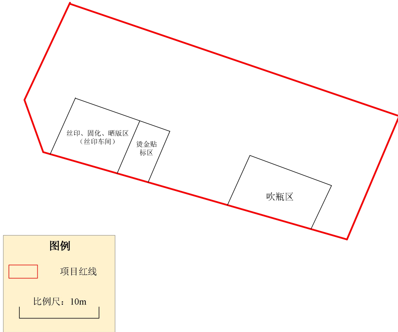
附图 4-5 4F 车间平面布置图
