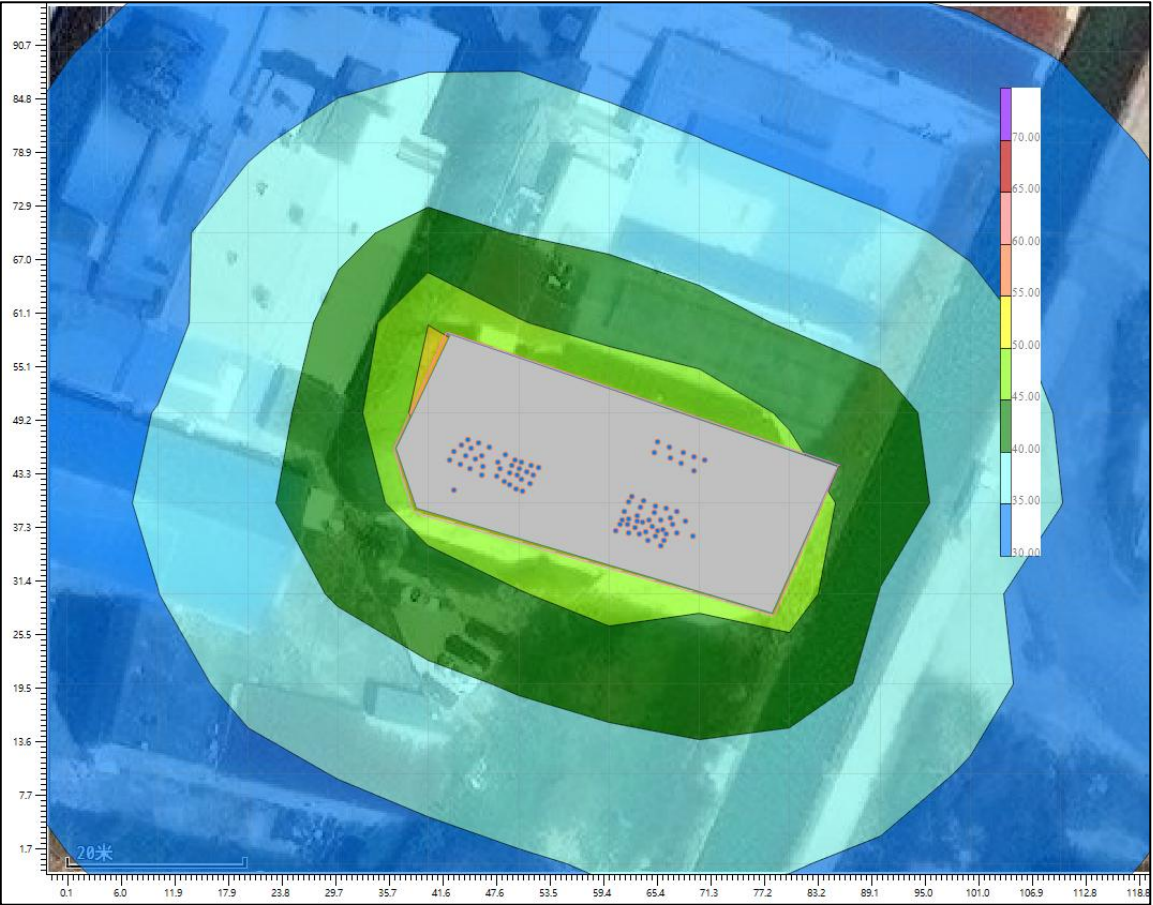
图 4-1 昼间噪声贡献值等值线示意图
