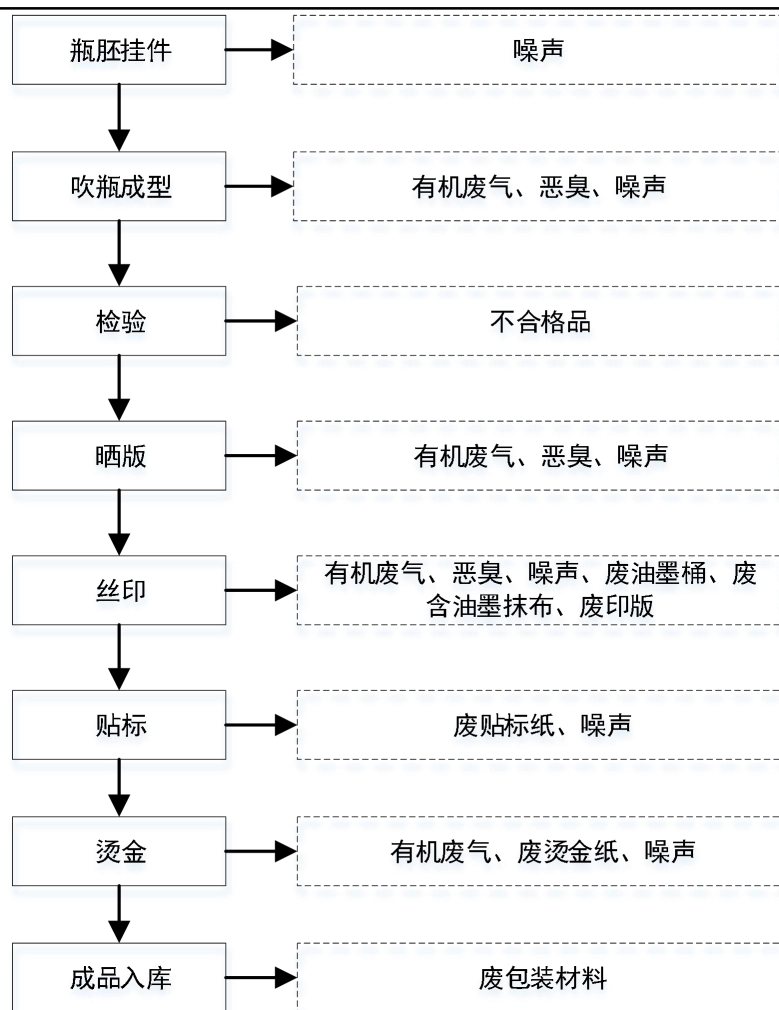
图 2-2 工艺流程及排污节点图
