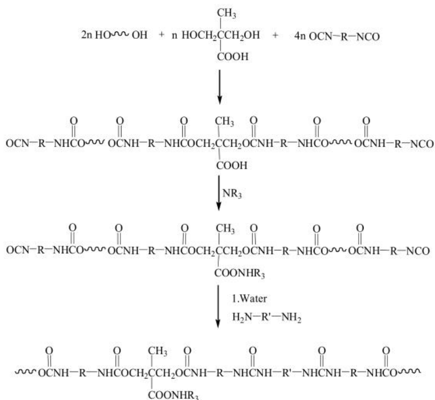
图 2-6 水性聚氨酯树脂的反应原理
