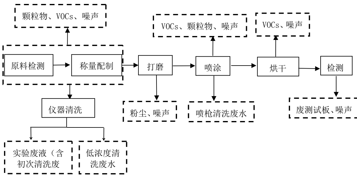
图 2-5 本扩建项目质量测试工艺流程及产污环节示意图
