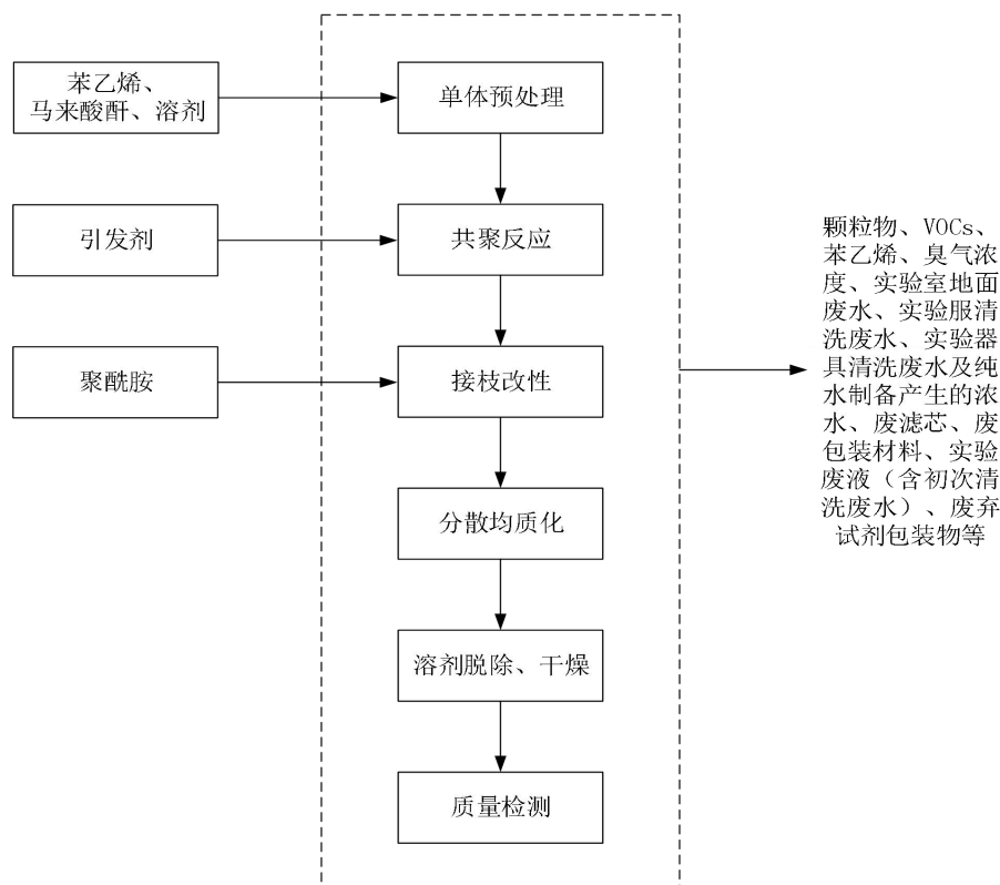
图 2-3 本扩建项目分散剂合成工艺流程及产污环节示意图
