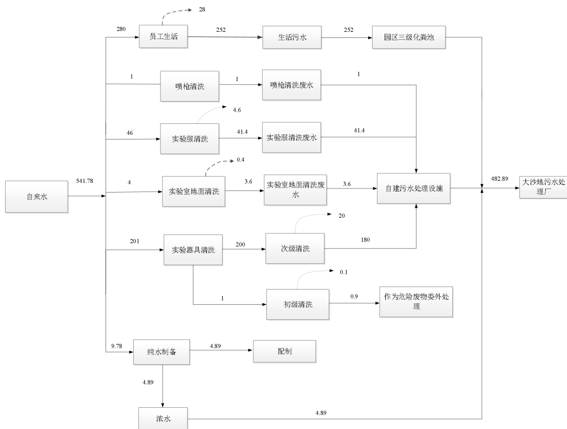
图 2-2 扩建后全厂水平衡图 (单位: m³/a)
