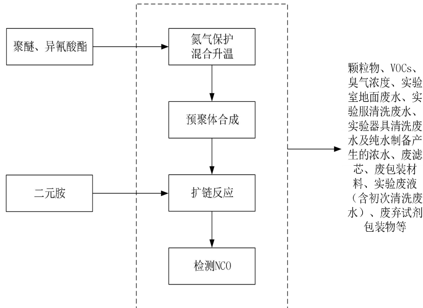
图 2-4 本扩建项目增稠剂合成工艺流程及产污环节示意图
