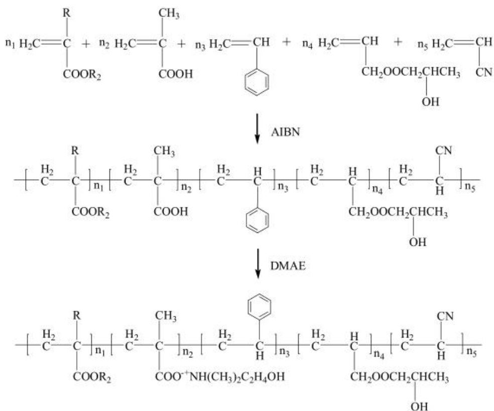
图 2-8 水性丙烯酸乳液的反应原理
