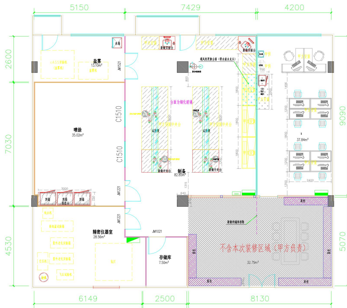
附图 3-1 项目 905-906 房平面布置图
