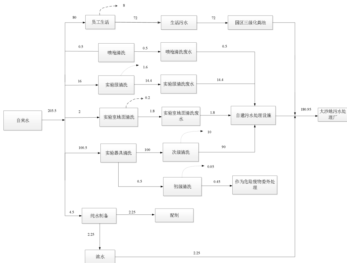
图 2-1 本扩建项目水平衡图 (单位: m³/a)
