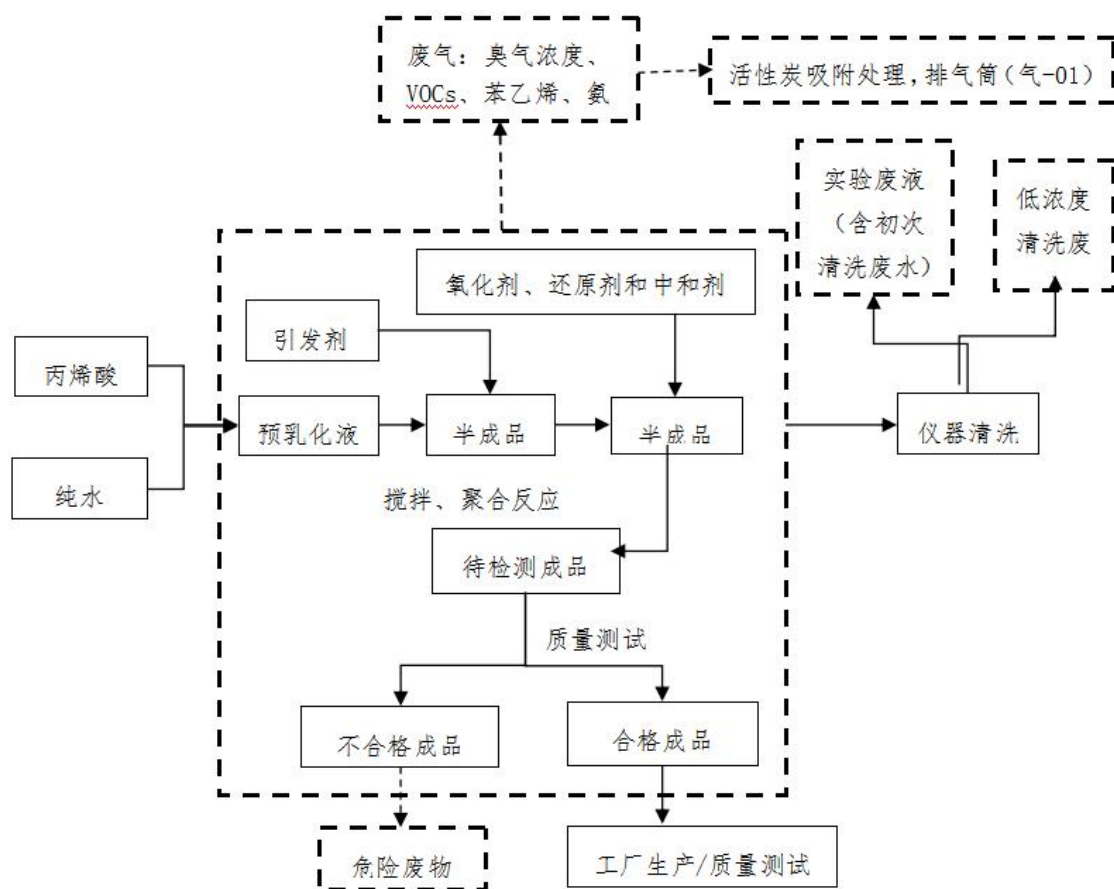
图 2-9 水性丙烯酸乳液研发工艺和产污环节图
