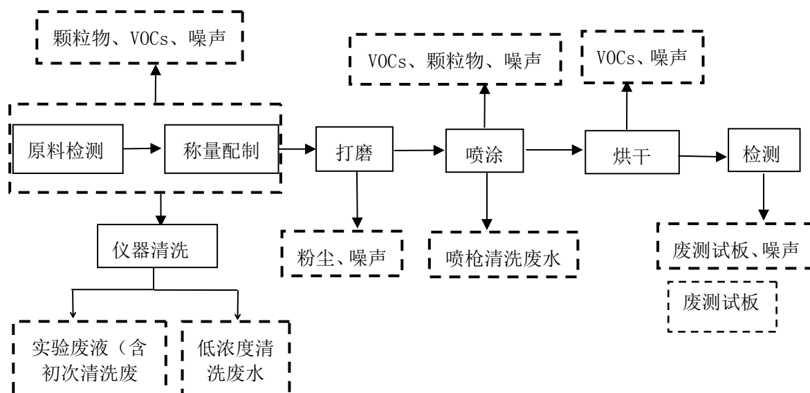
图 2-10 质量测试工艺和产污环节图
