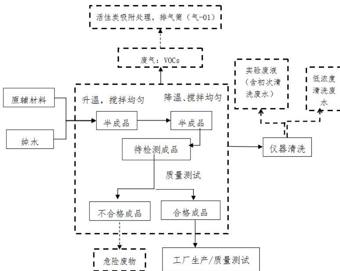
图 2-7 水性聚氨酯树脂研发工艺和产污环节图
