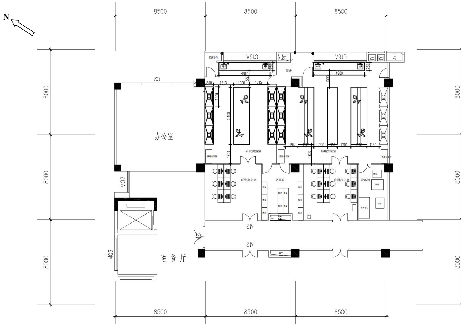
附图3-2项目907-908房平面布置图
