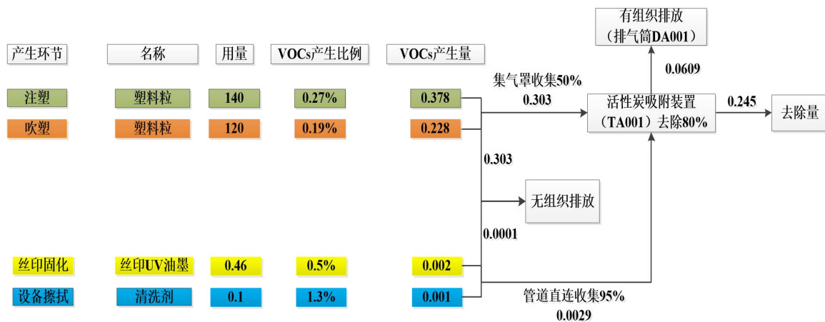
图 2-2 本项目 VOCs 平衡图 (单位 t/a)
