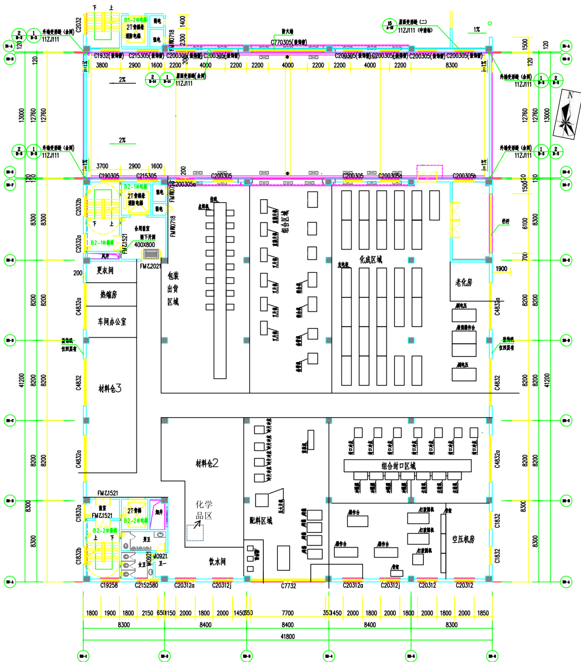
第 5 层平面布置图 附图 3 项目平面布置图
