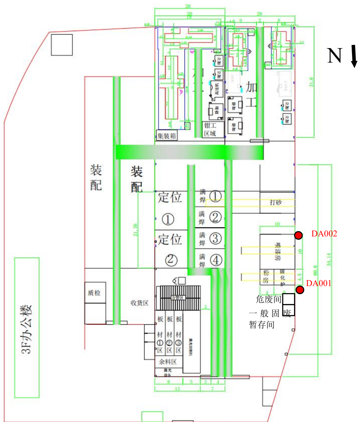
附图5 项目总平面布置图
