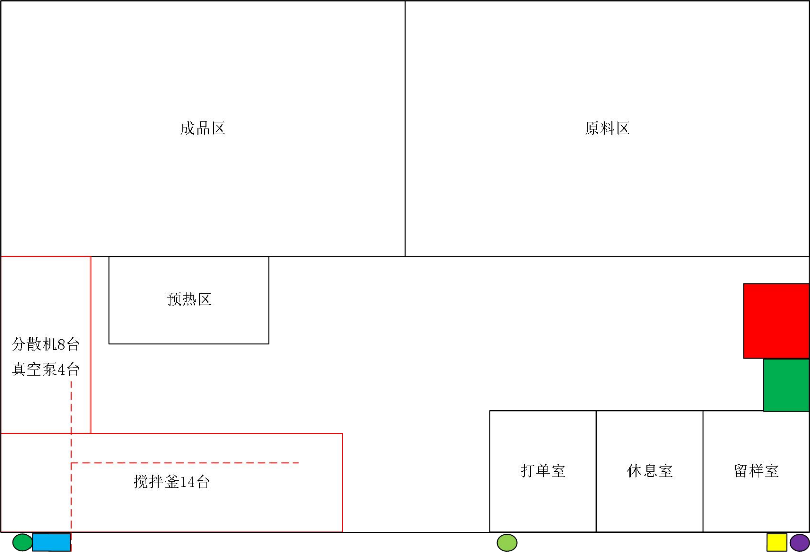
附图4 建设项目车间平面布局图
