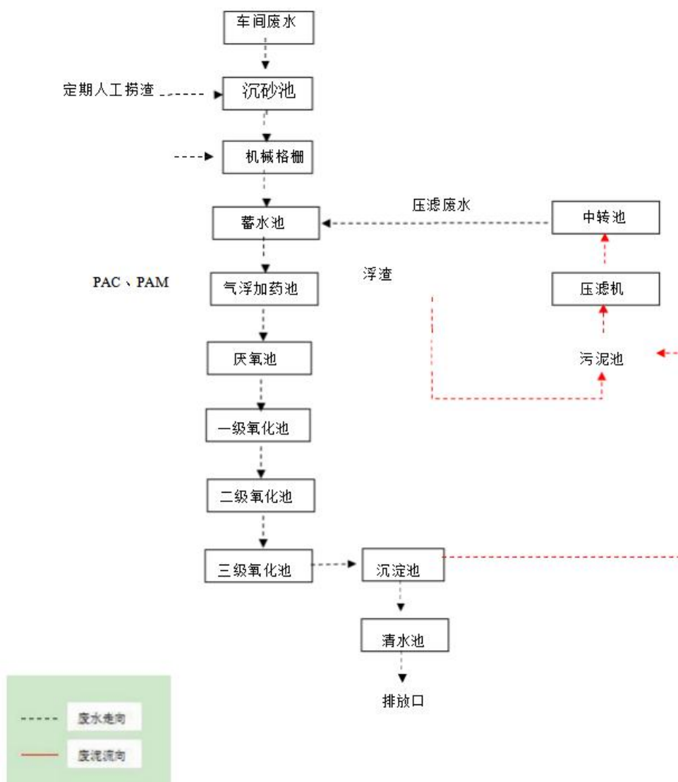
图 4-1 生产废水处理工艺流程
