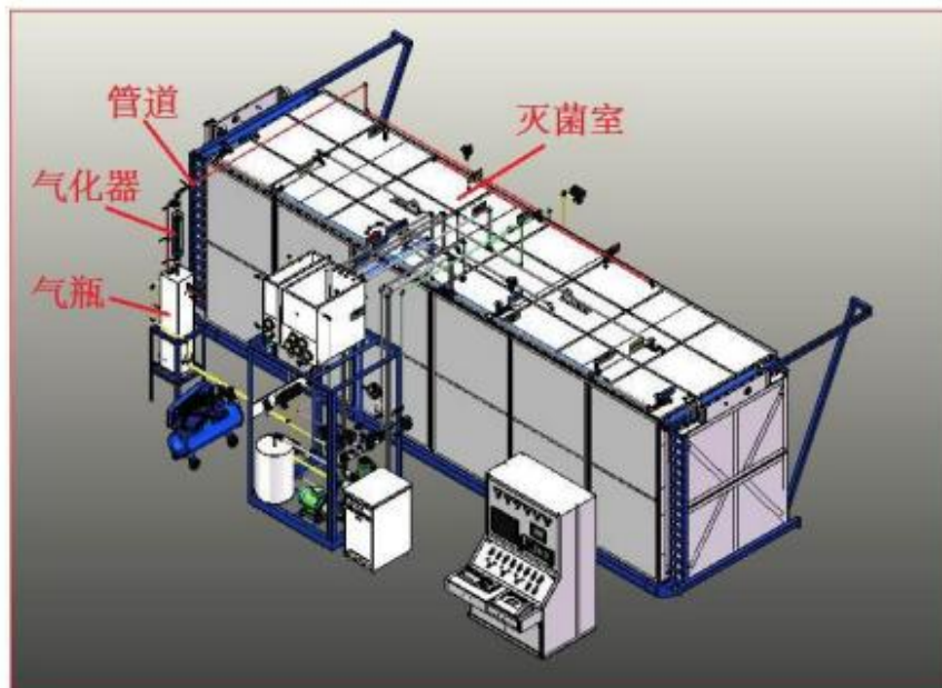
图2-7环氧乙烷灭菌柜图
