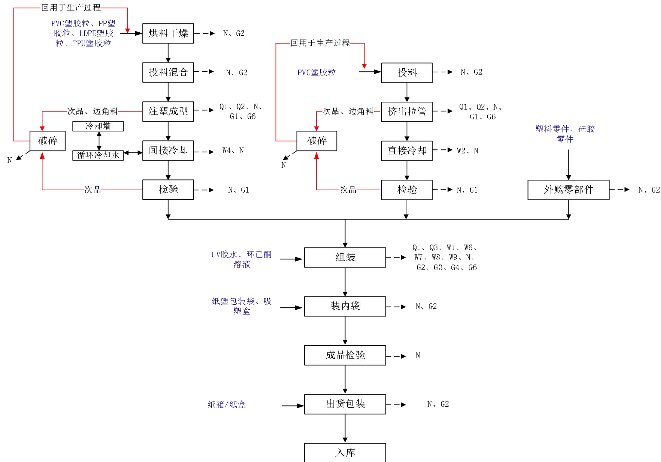
图2-4 本项目生产工艺流程图2
