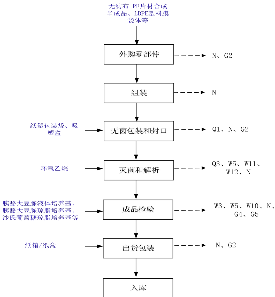
图 2-5 本项目生产工艺流程图
