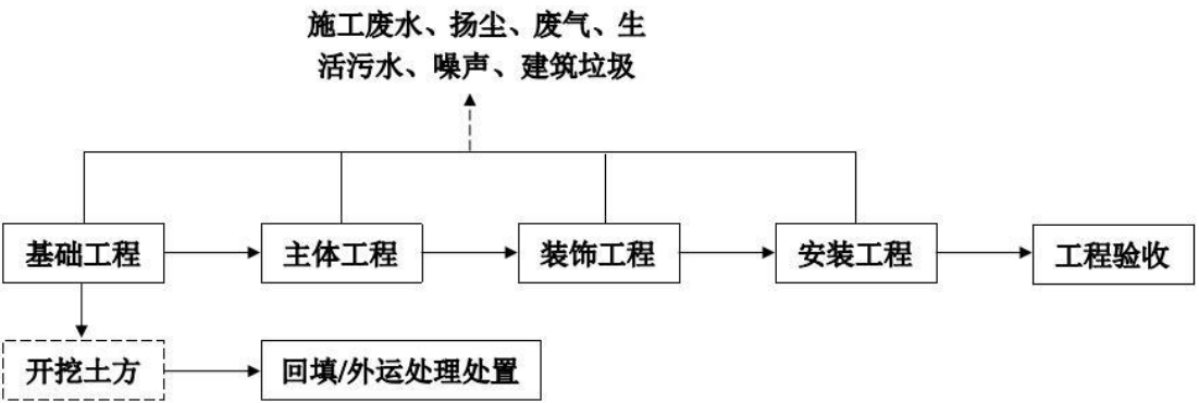
图2-2施工期工艺流程及产污环节图
