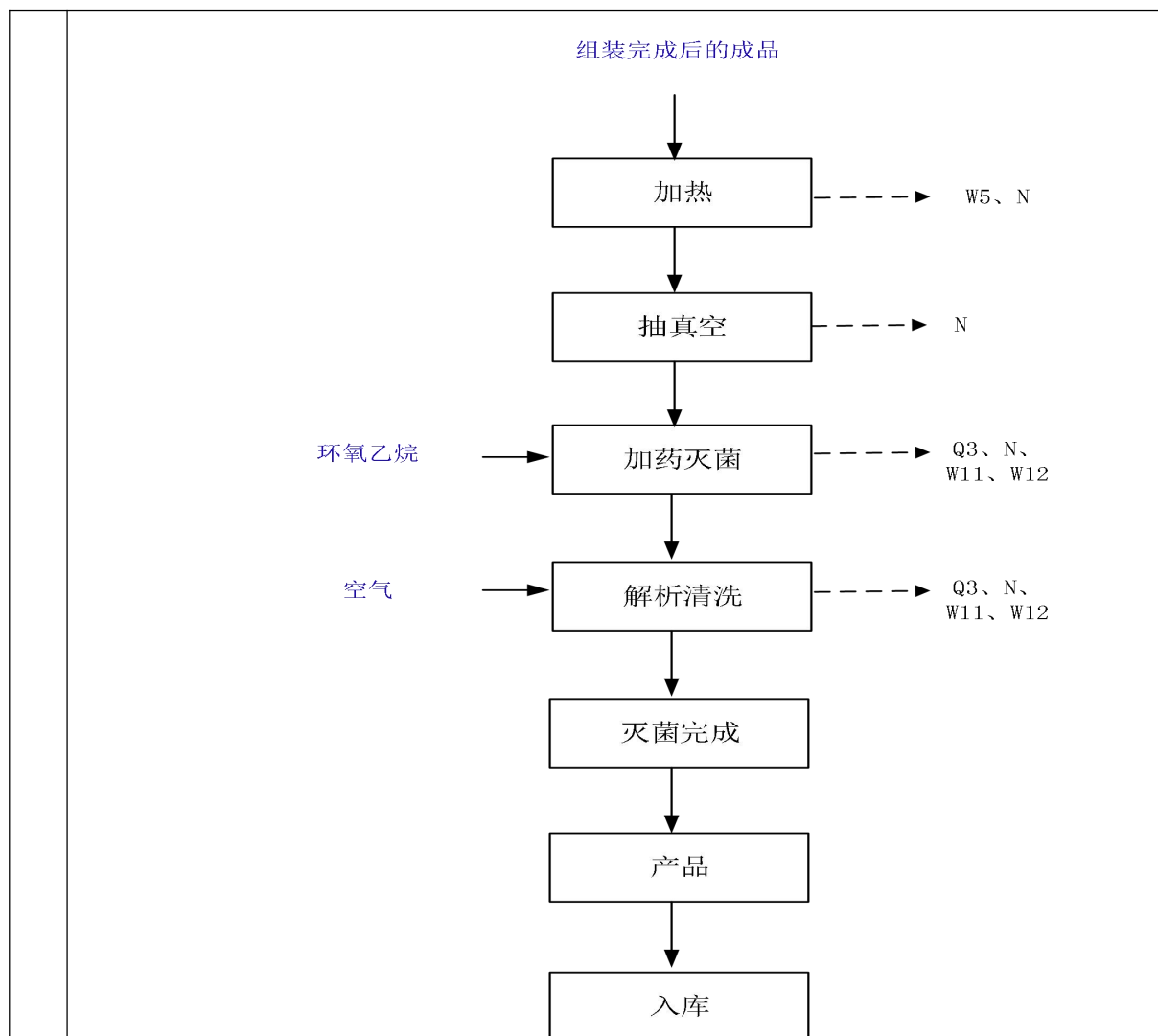
图2-6灭菌工艺流程及产污节点图3
