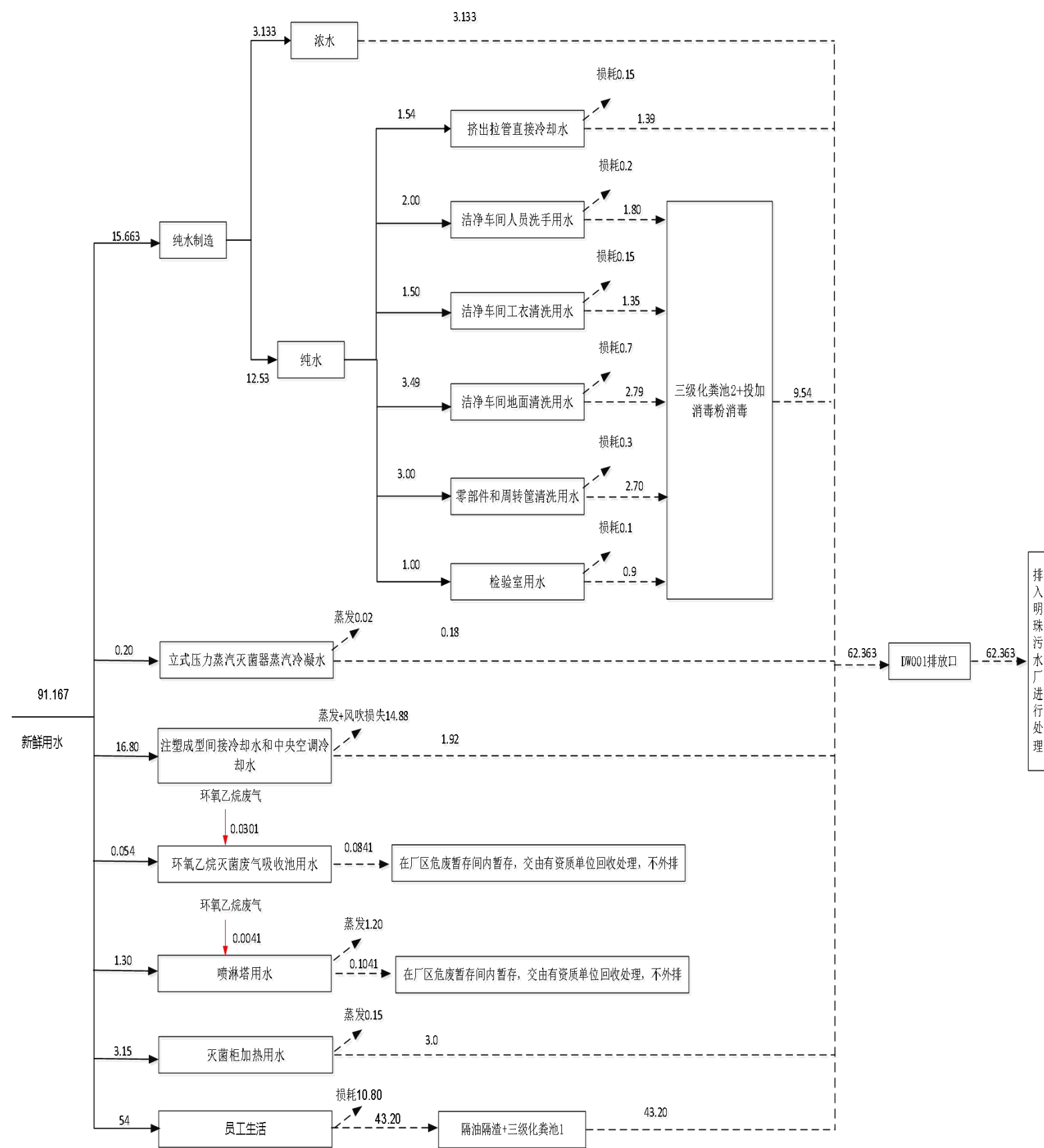
图2-1 本项目水平衡图 (单位t/d)
