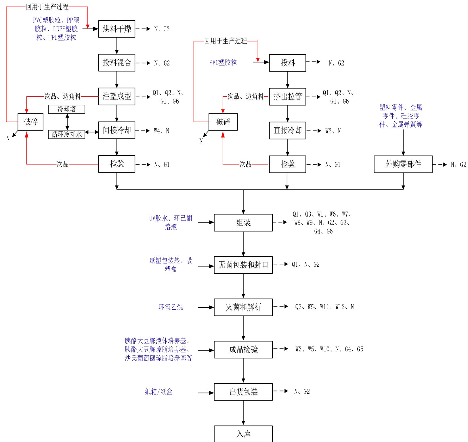
图2-3 本项目生产工艺流程图1
