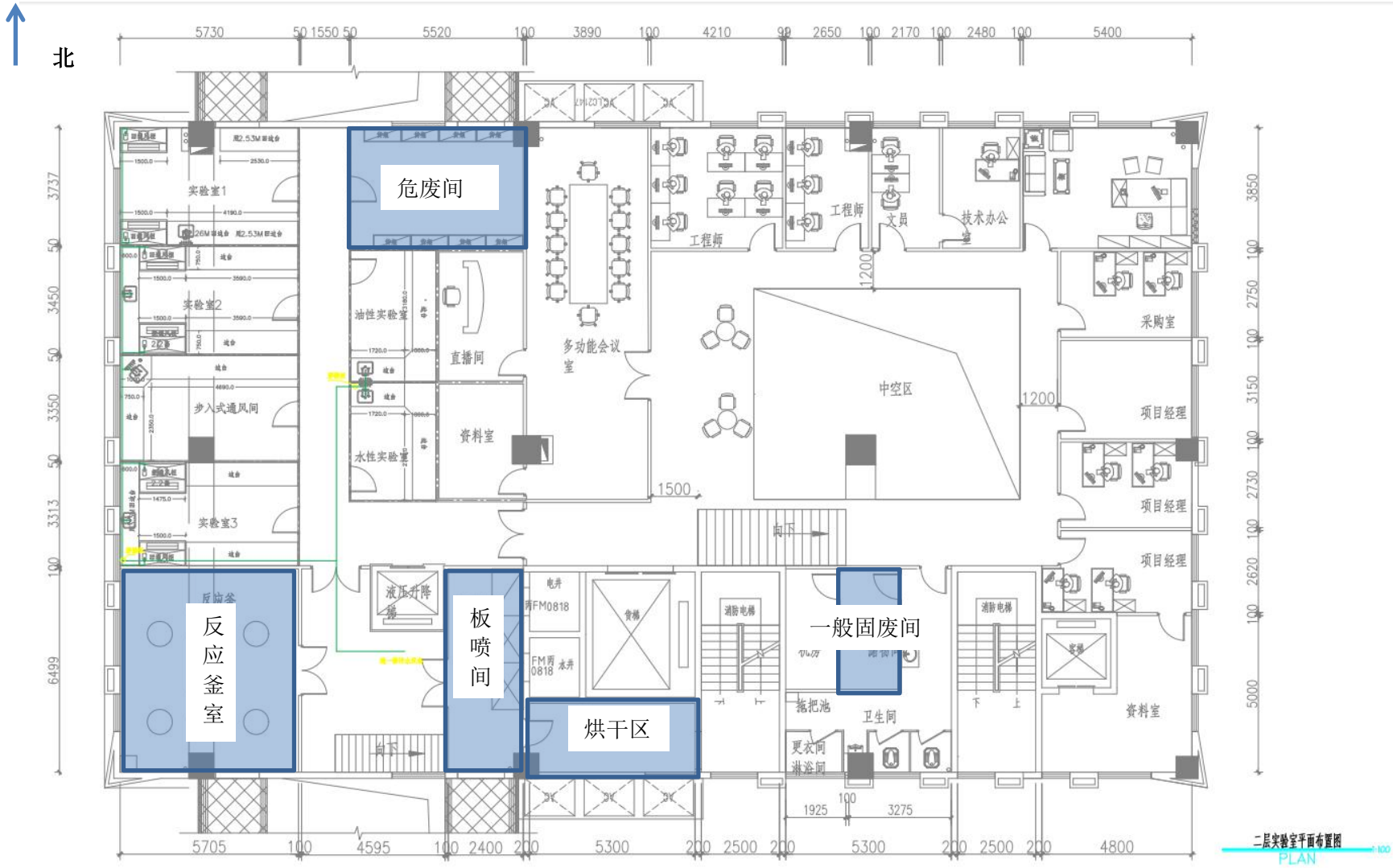
附图 3-2 建设项目平面布置图（2F）
