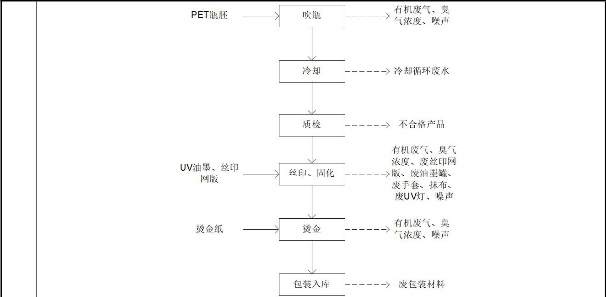
图 2-3 塑料瓶吹瓶的工艺流程
