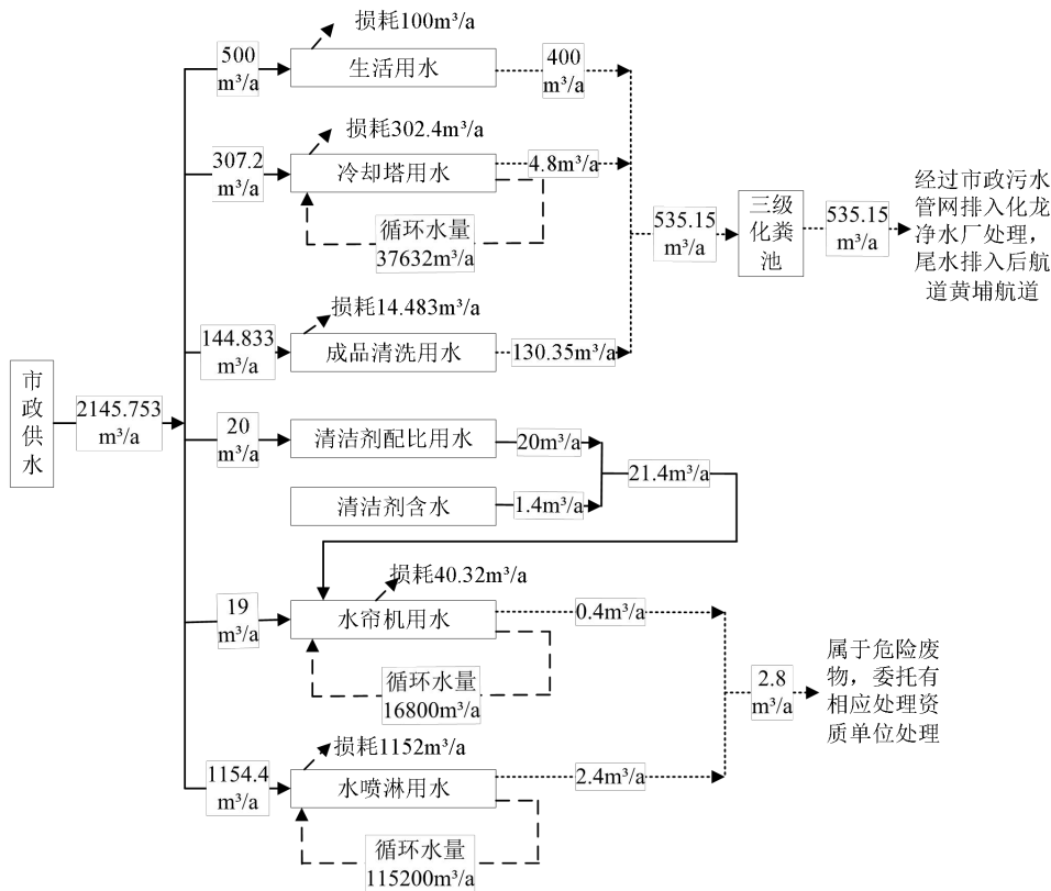
图 2-2 水平衡图
