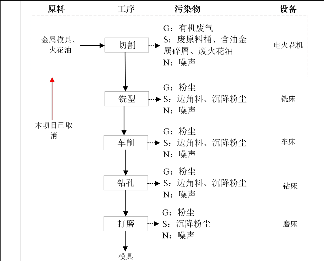
图 2-7 原项目模具加工工艺流程及产污节点图
