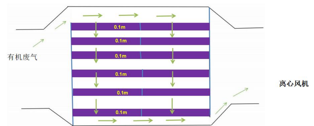
图 4-5 活性炭箱设计示意图
