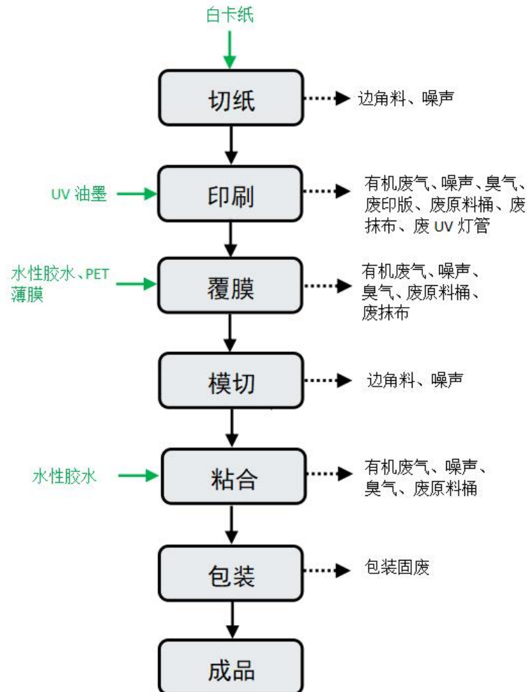
图 2-2 化妆品彩盒生产工艺流程及产污环节图
