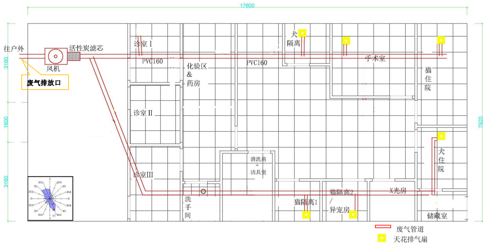
附图 4-2 院区废气管道平面布置图
