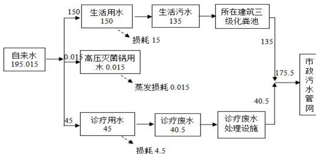
图 2-3 扩建后全院水平衡图（单位：m³/a）
