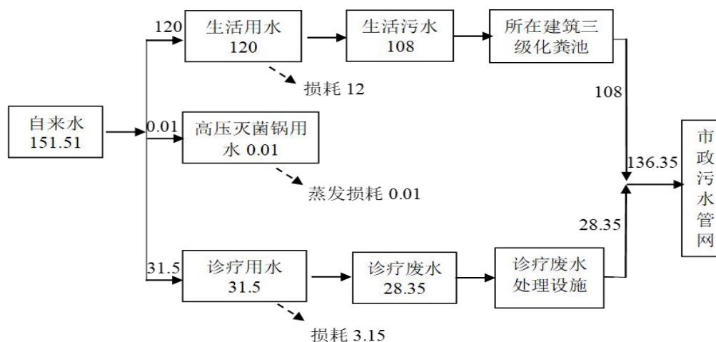
图 2-1 现有项目水平衡图（单位：m 3 /a）
