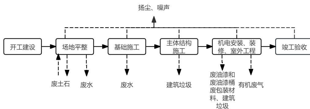
图2-2施工期工艺流程图
