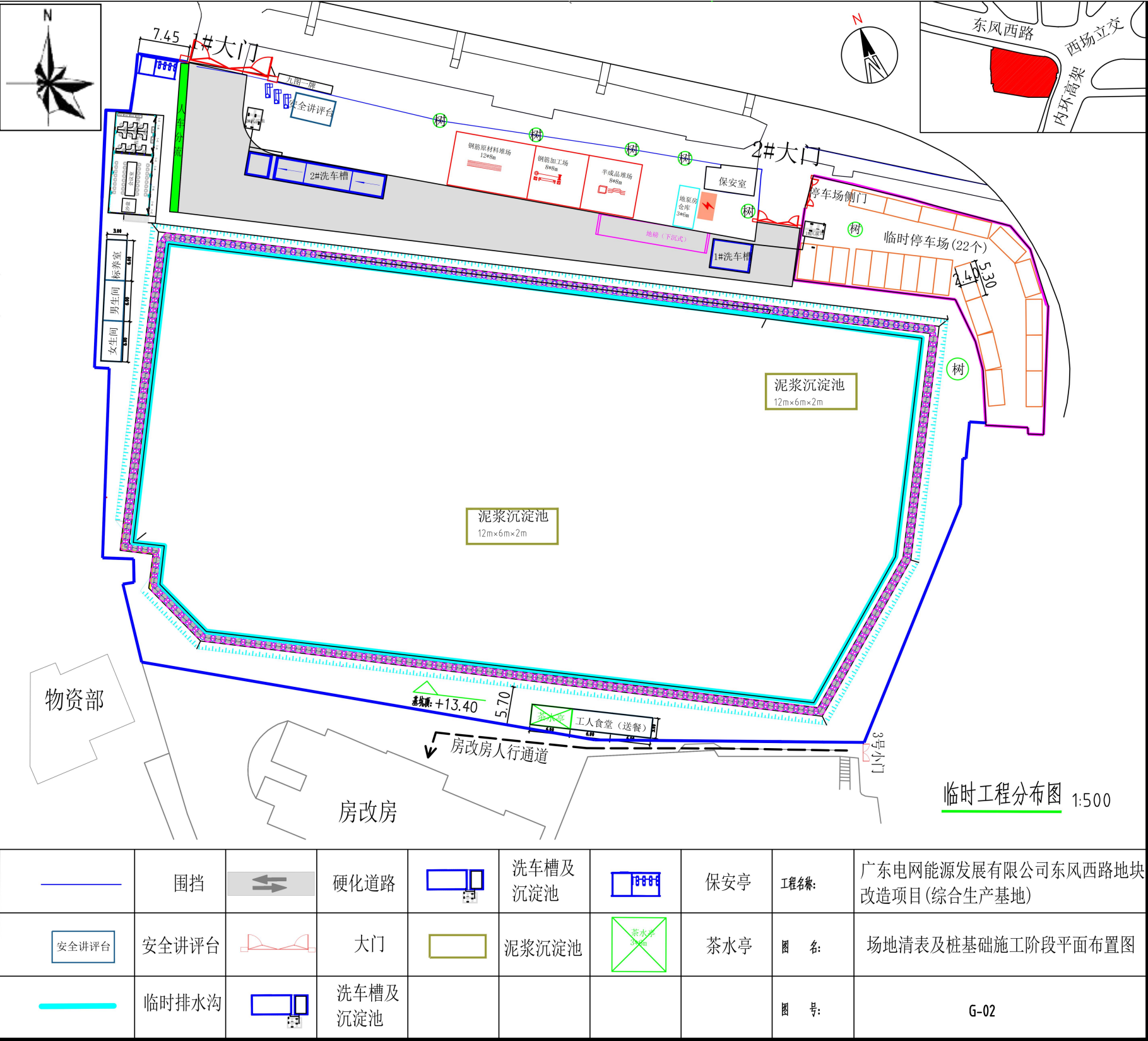
附图 29 临时工程分布图
