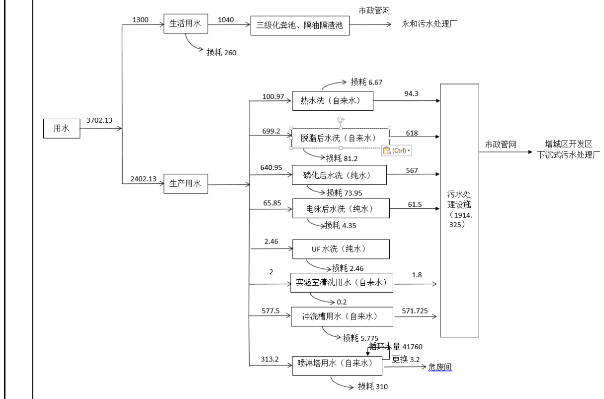
图 2-1 近期水平衡图 (t/a)
