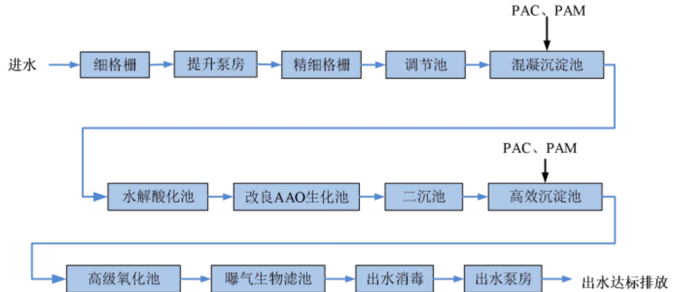
图 4-2 工业废水处理总体工艺路线图
