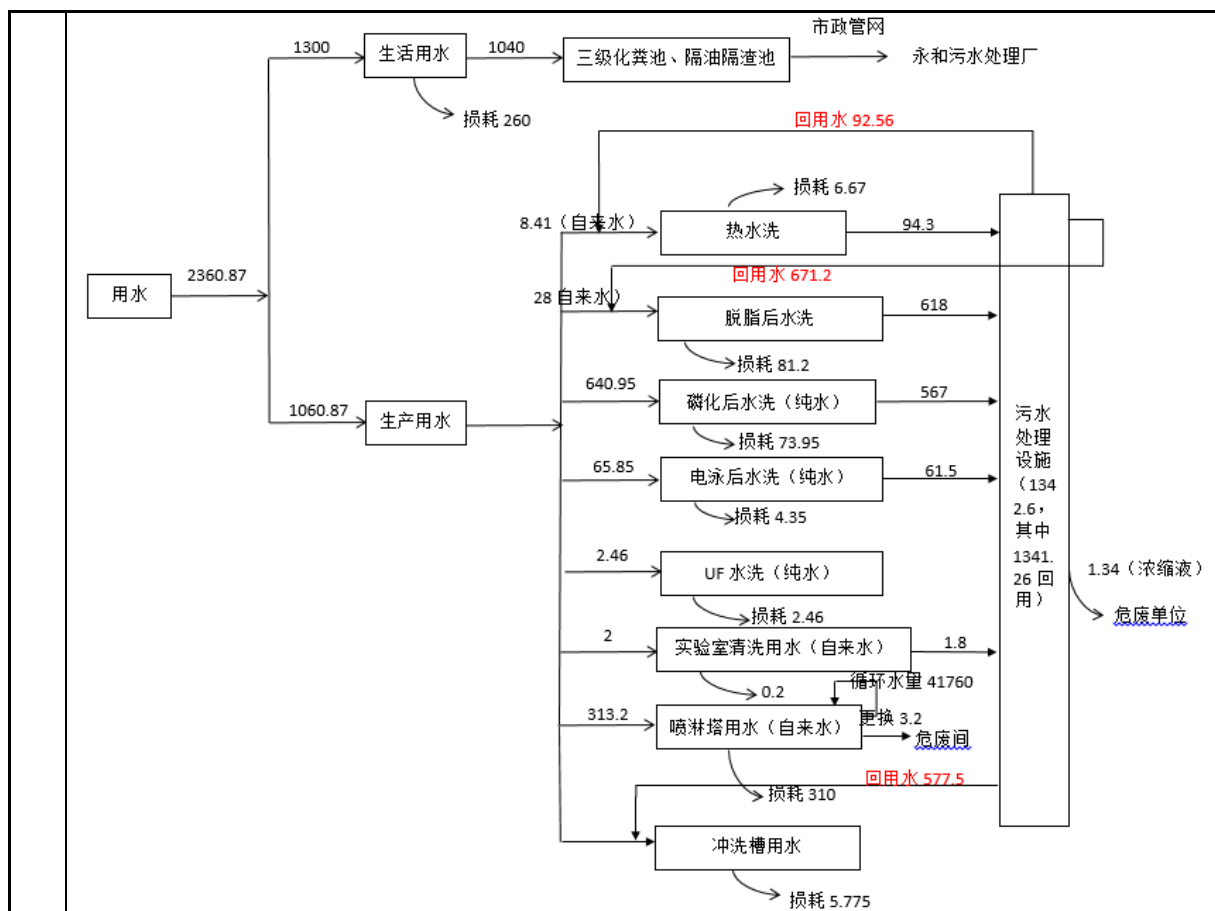
图 2-1 近期水平衡图 (t/a)
