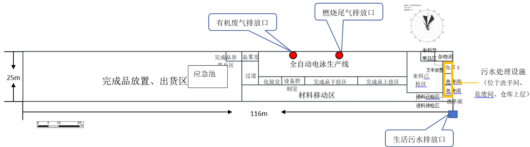
附图 2-1 平面布置图（电泳车间）
