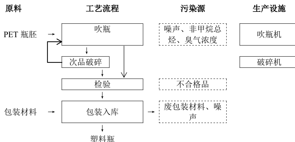
图 2-3 未批先建投产项目工艺流程及产污节点图
