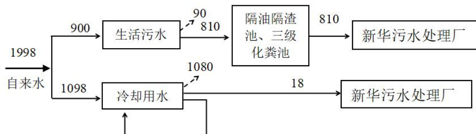
图 2-2 本项目水平衡图（单位 m³/a）
