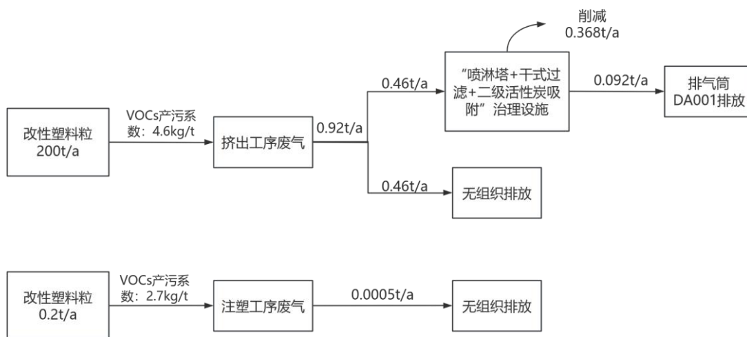
图 2-2 本项目 VOCs 平衡图
