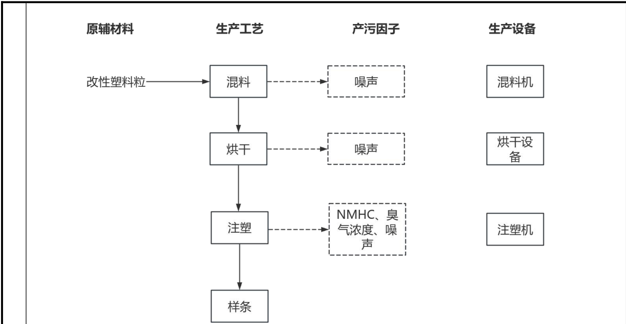
图 2-4 本项目试样注塑生产工艺流程及产污环节图
