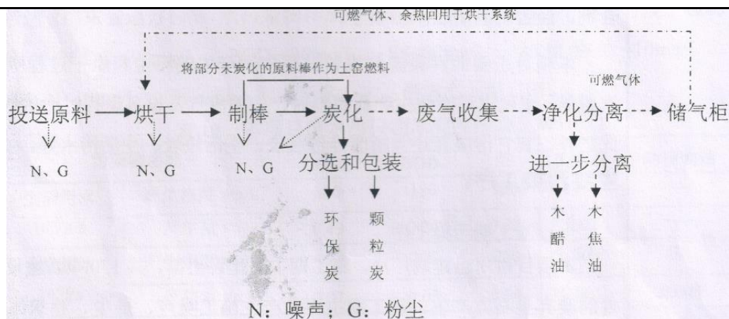
图 2-2 现有工程生产工艺流程图
