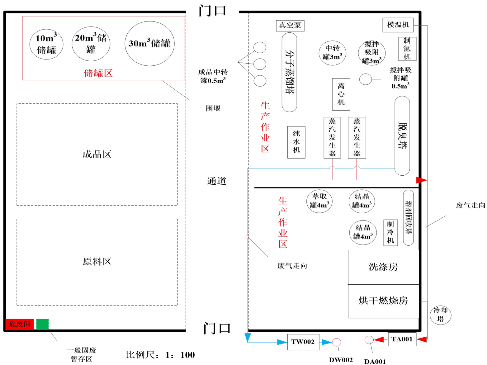
附图 4 建设目总平面布图
