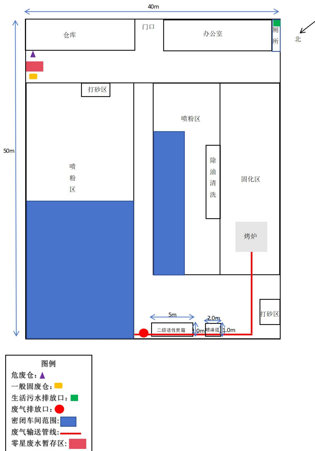
附图 4 项目平面布置图
