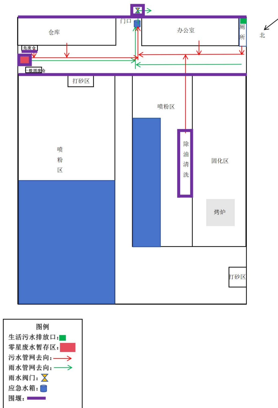
附图 4-1 项目雨污水及事故废水收集系统图
