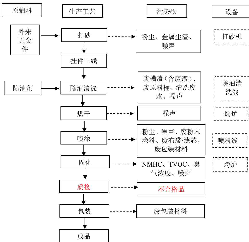
图 2-2 工艺流程及产污节点图
