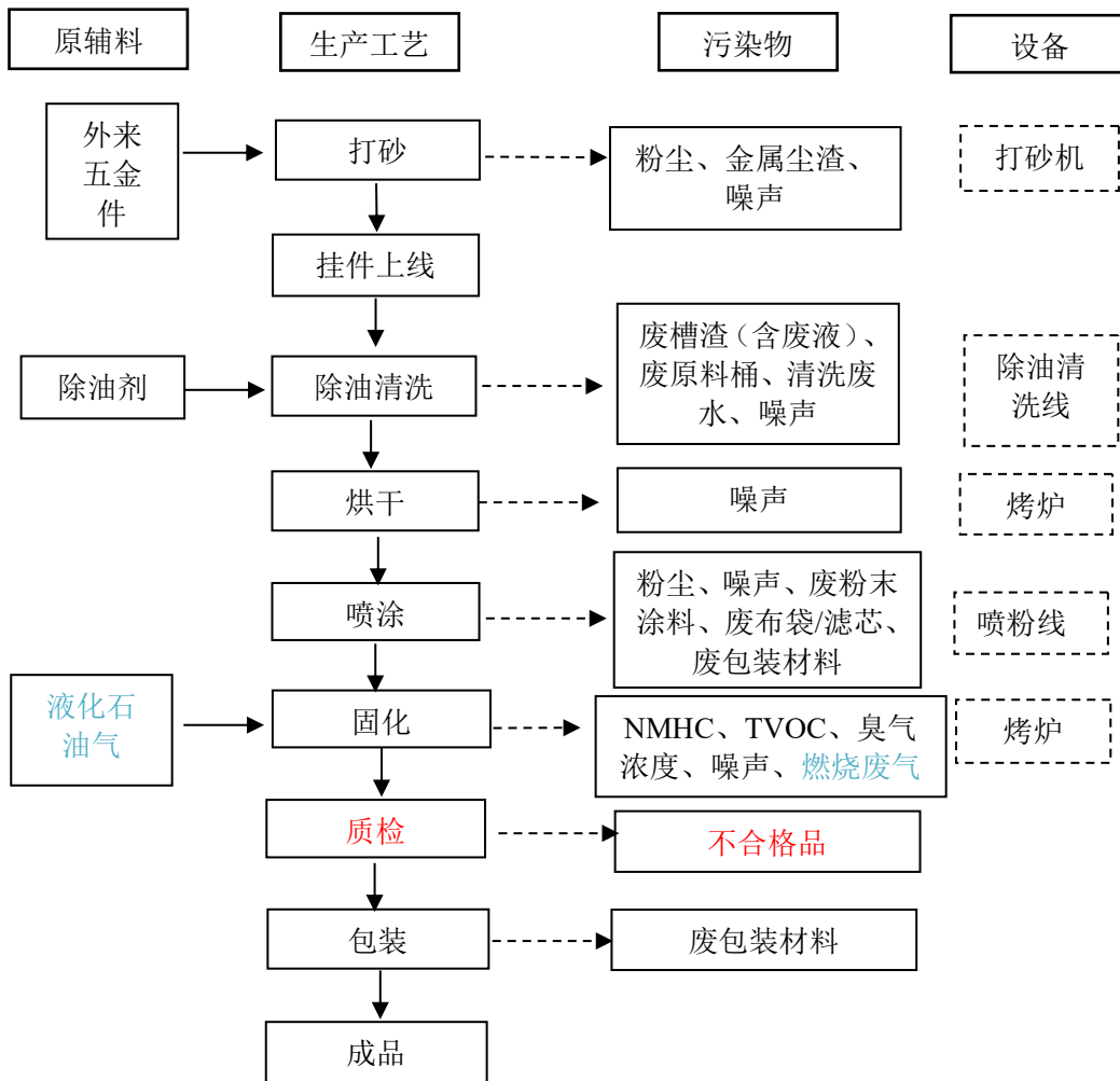
图 2-3 项目工艺流程及产污节点图
