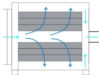
图 4-1 一级活性炭吸附装置示意图
