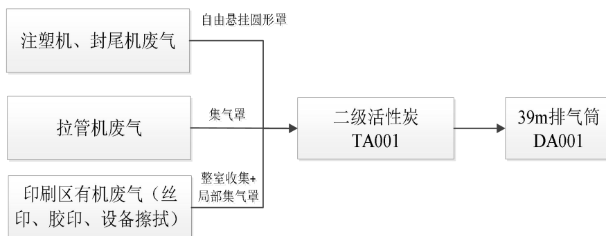
图 4-2 本项目废气处理工艺流程示意图
