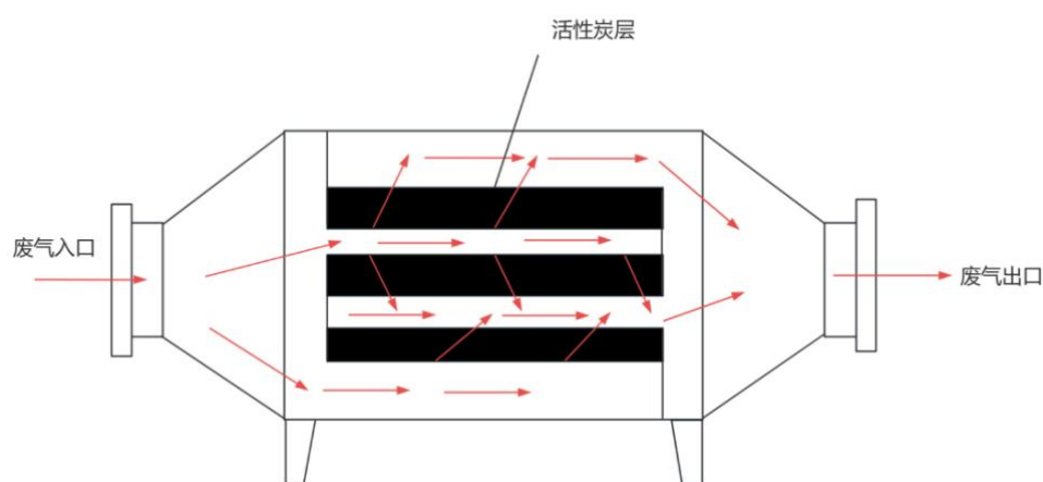
图 4-5 本项目活性炭箱设计图（红色箭头为废气走向）
