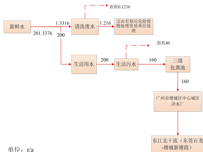
图 2-1 项目水平衡图
