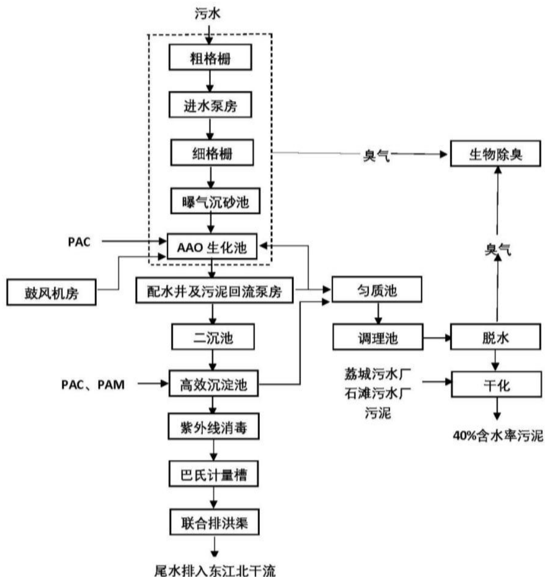
图 4-2 中心城区净水厂工艺流程图
