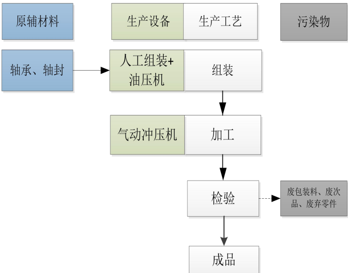
图2-3电控阀生产工艺流程图
