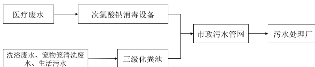
图 4-1 运营期间废水处理措施
