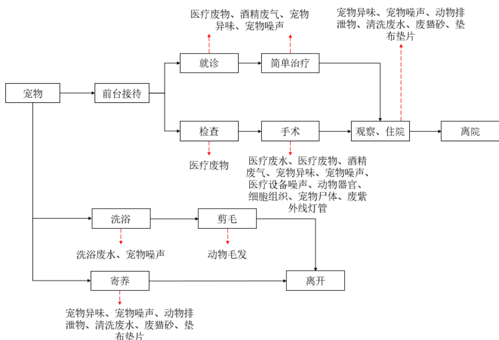
图 2-2 宠物诊疗、美容流程产污示意图
