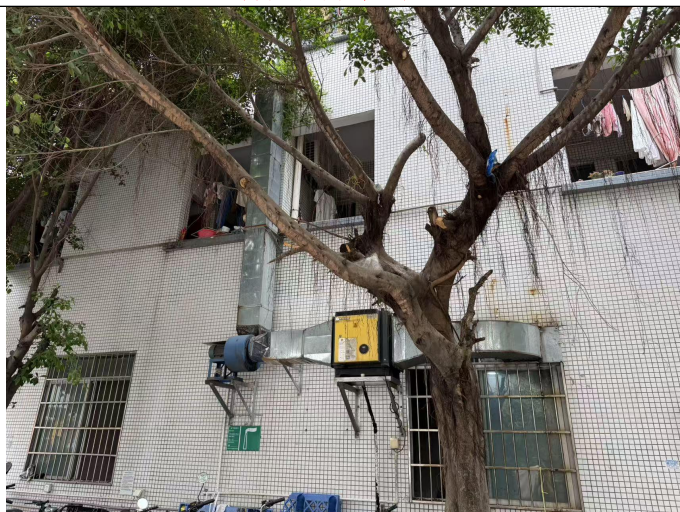
活性炭吸附装置
