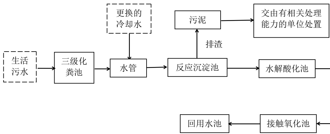
图 4-2 项目一体化污水处理工艺流程图
