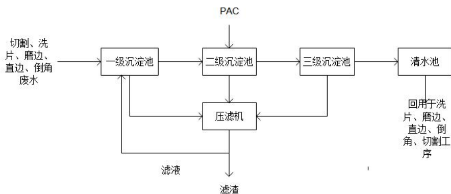
图 4-1 污水处理设施处理流程
