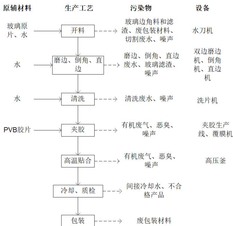
图 2-2 夹胶玻璃生产工艺流程
