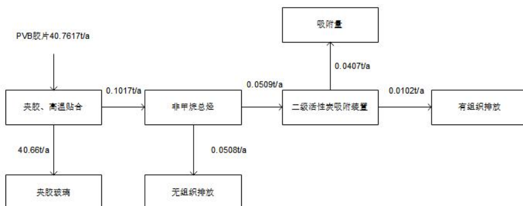
图 4-2 项目有机废气平衡图
