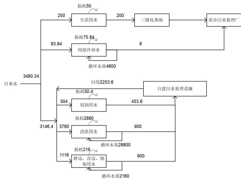
图 2-1 项目水平衡图 (t/a)
