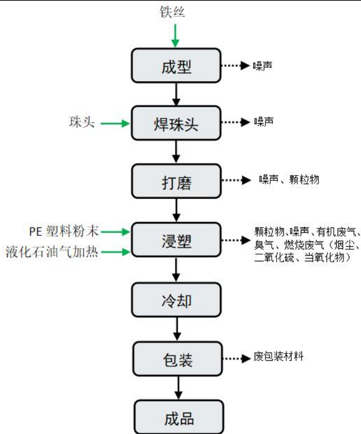
图2-2 衣架生产工艺流程图
