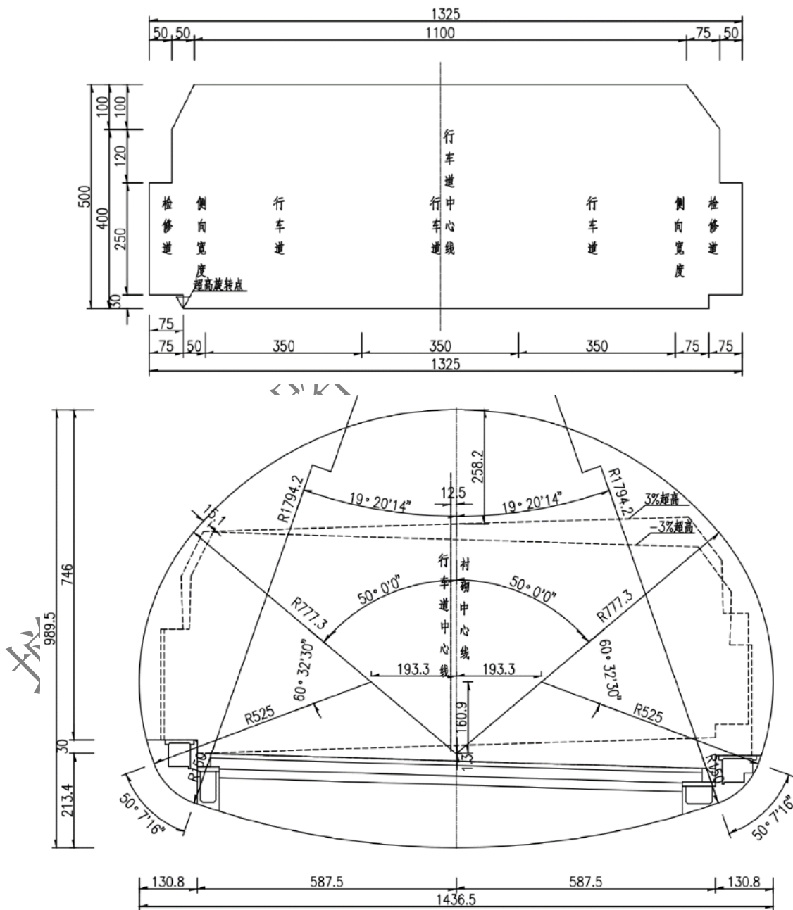
图 3.1-7 分离式隧道建筑限界及内轮廓图
