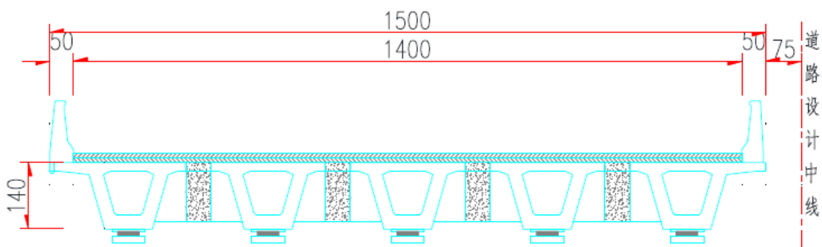
图 3.1-6 古郎山塘大桥标准横断面（无人非道）
