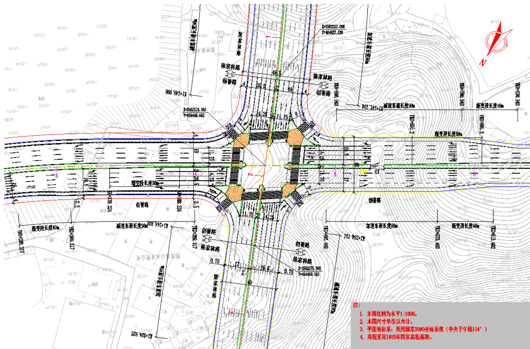
图 3.1-11 项目平面交叉布置图
