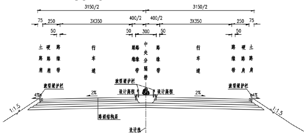
图 3.1-3 YK0+449.798~YK0+920 段整体式路基横断面图
