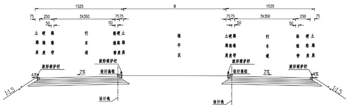
图 3.1-4 YK0+920~YK1+125 段分离式路基横断面图
