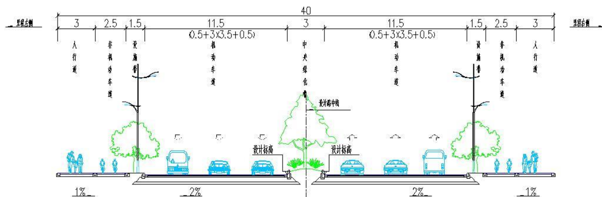
图 3.1-1 现状增科路横断面图
