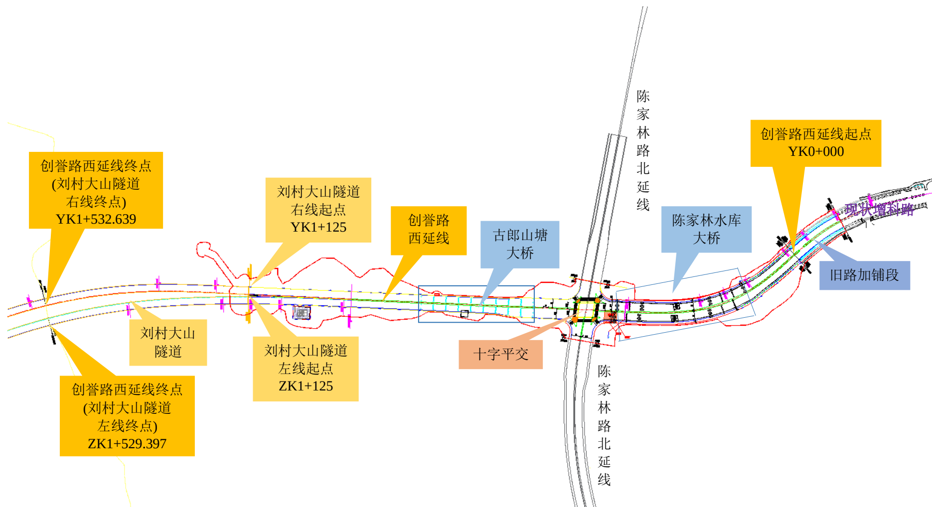
图 3.1-10 项目路线及主要相交道路平面布置图
