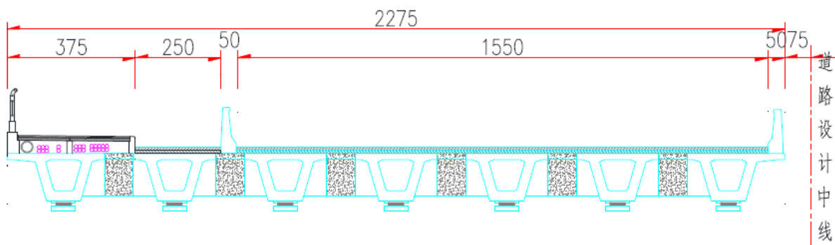
图 3.1-5 陈家林水库大桥标准横断面（有人非道）
