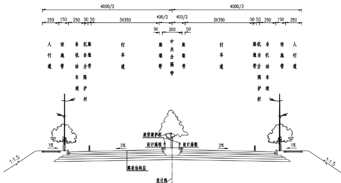
图 3.1-2 起点至陈家林路段（YK0+000~YK0+449.798）整体式路基横断面图
