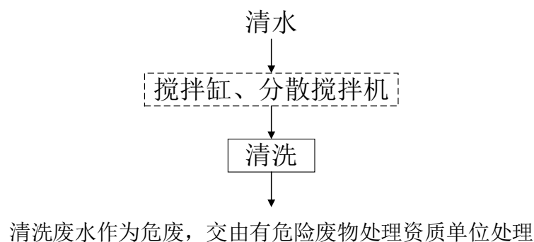
图 2-3 项目洗缸工艺流程图
