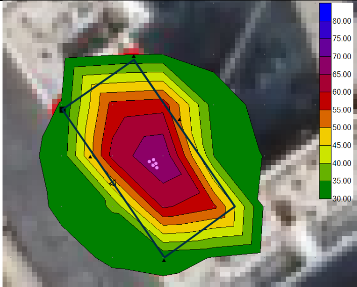
图 4-1 主要噪声源分布及贡献值预测图
