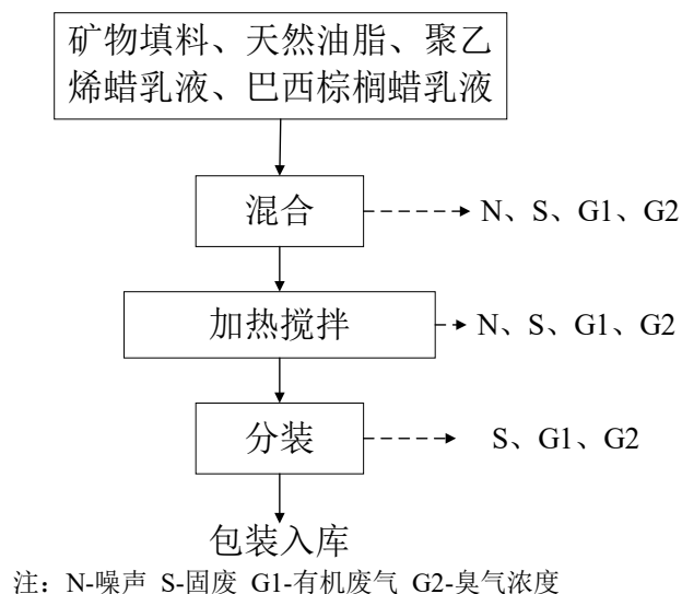
图 2-3 项目蜡块生产工艺流程图
